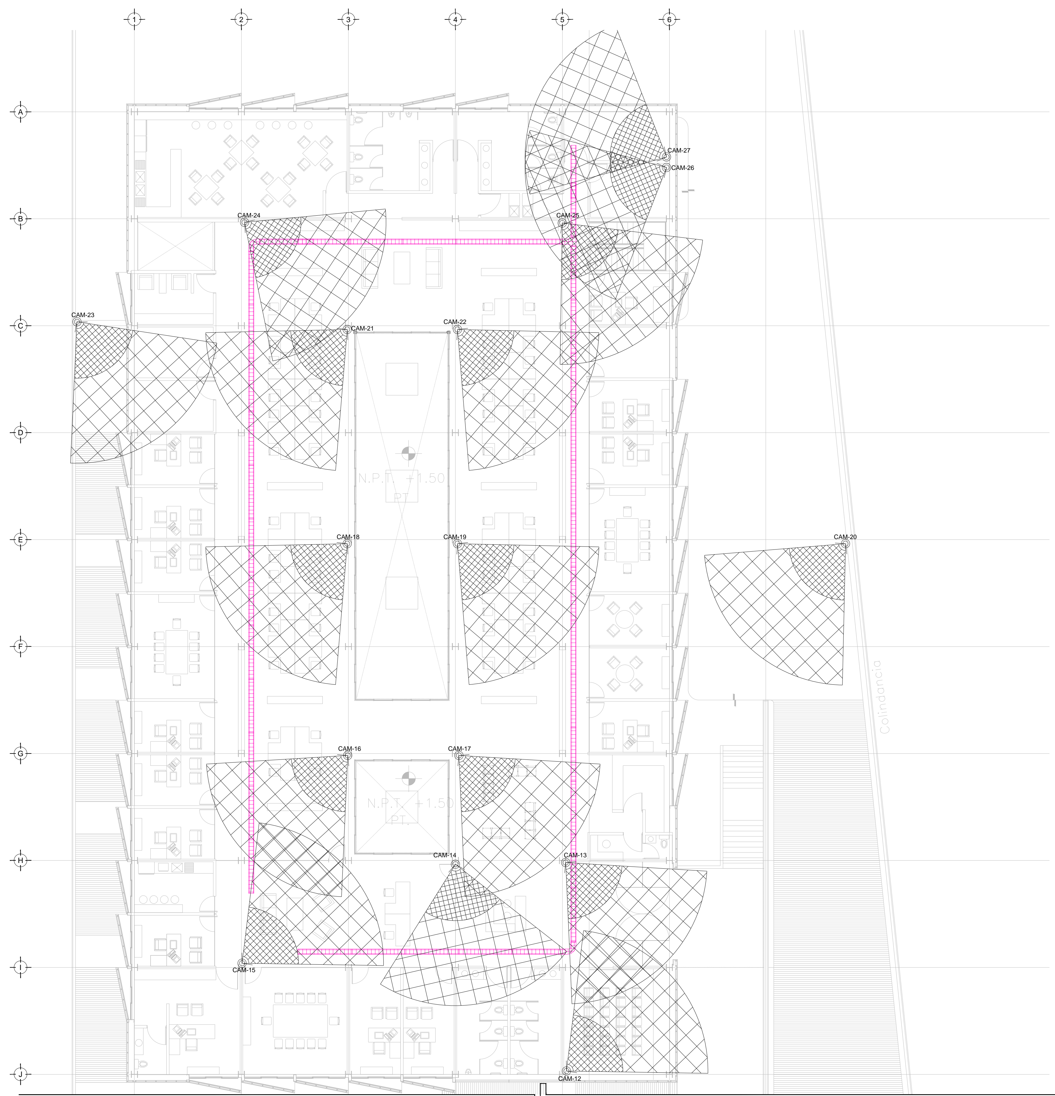
TENDIDO DE INSTALACIÓN CCTV (DELEGACION). N.P.T +1.50 mts. ESC: 1:125
