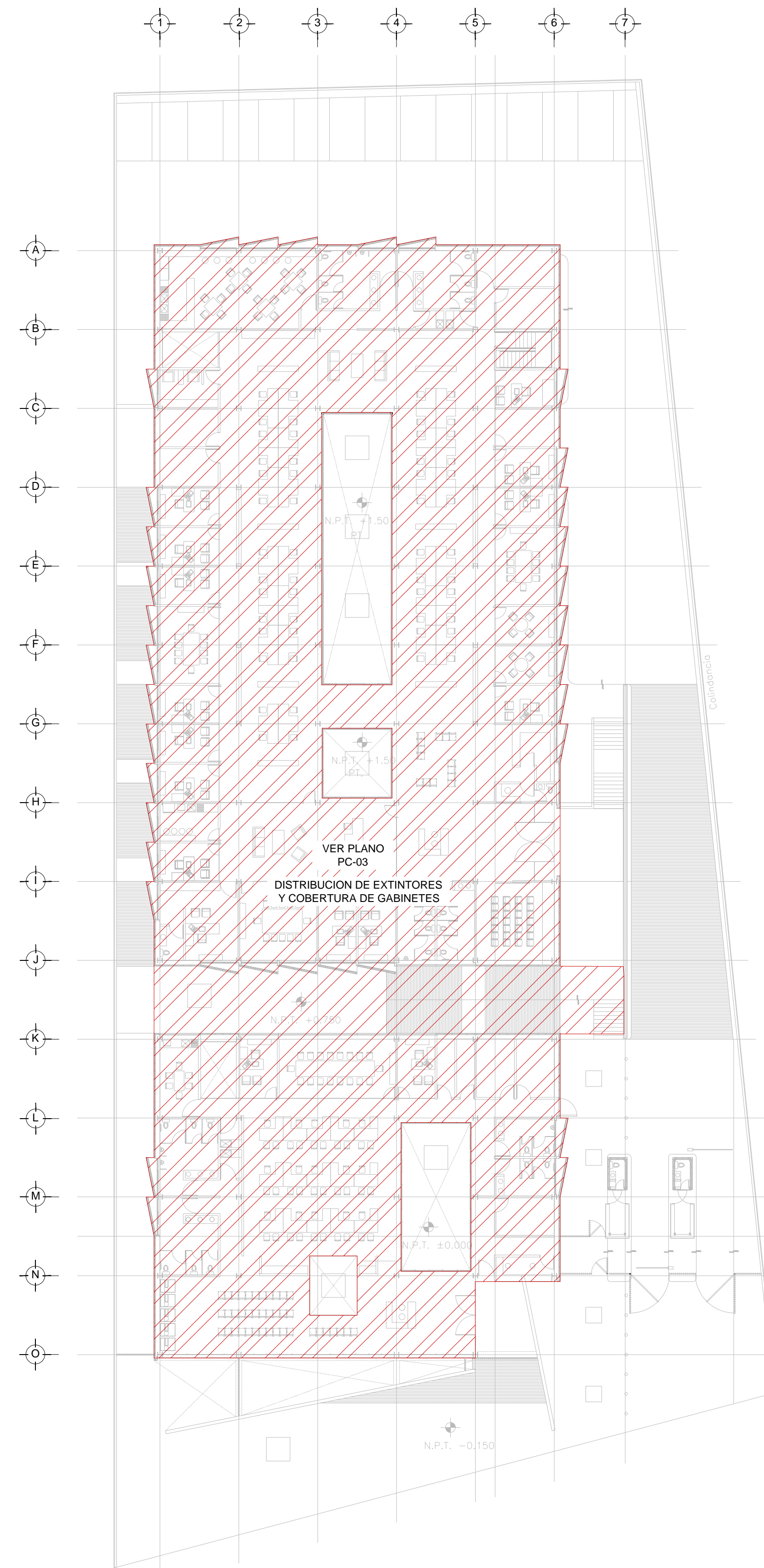
PLANTA BAJA CESIS - NIVEL 0.00 Y +1.50 ESC. 1:250
