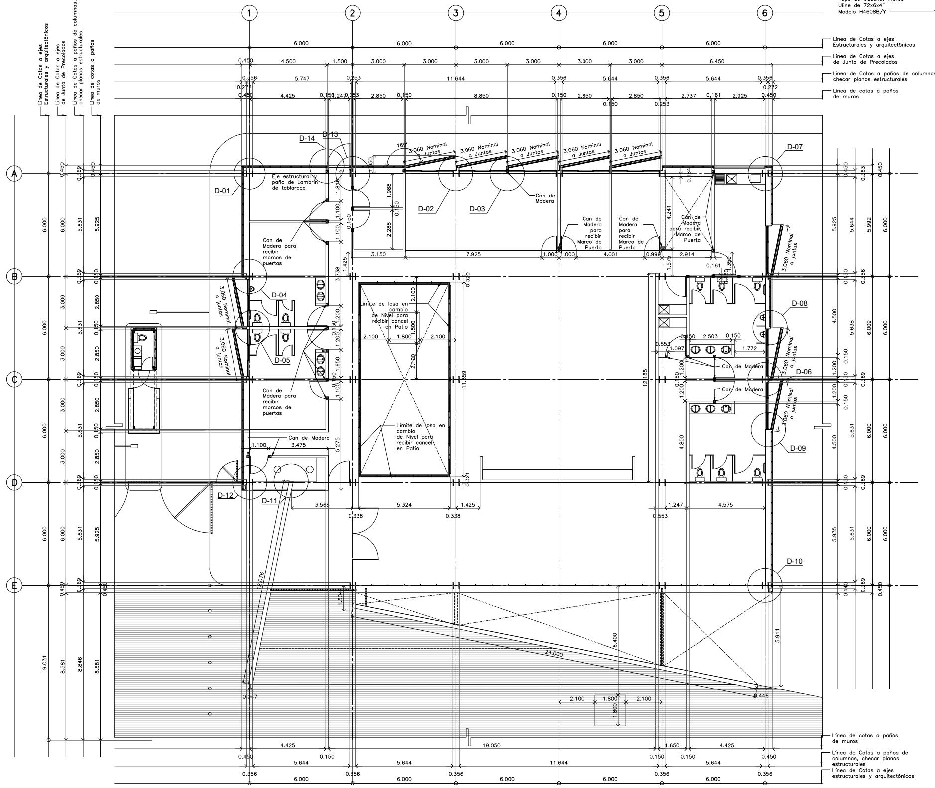
DETALLE-01 PLANTA ARQUITECTÓNICA DE ALBAÑILERÍA NIVEL ±0.000
