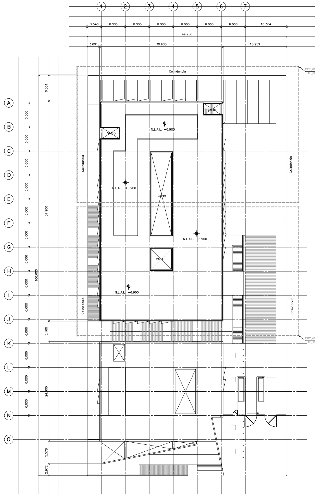
PLANTA DE AZOTEA DELEGACIÓN NIVEL +6.900
