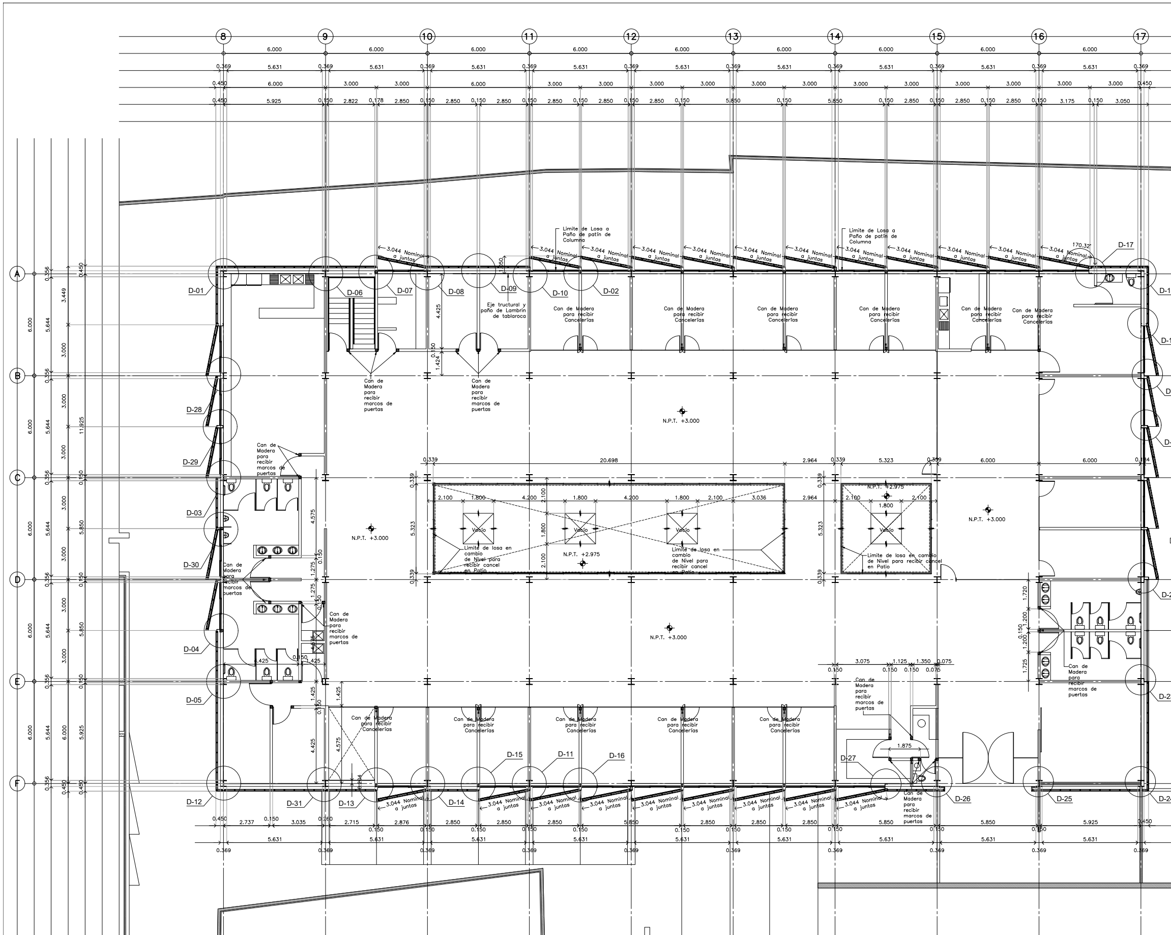
PLANTA ARQUITECTÓNICA ALBAÑILERIAS NIVEL + 3.000 DETALLE 04
