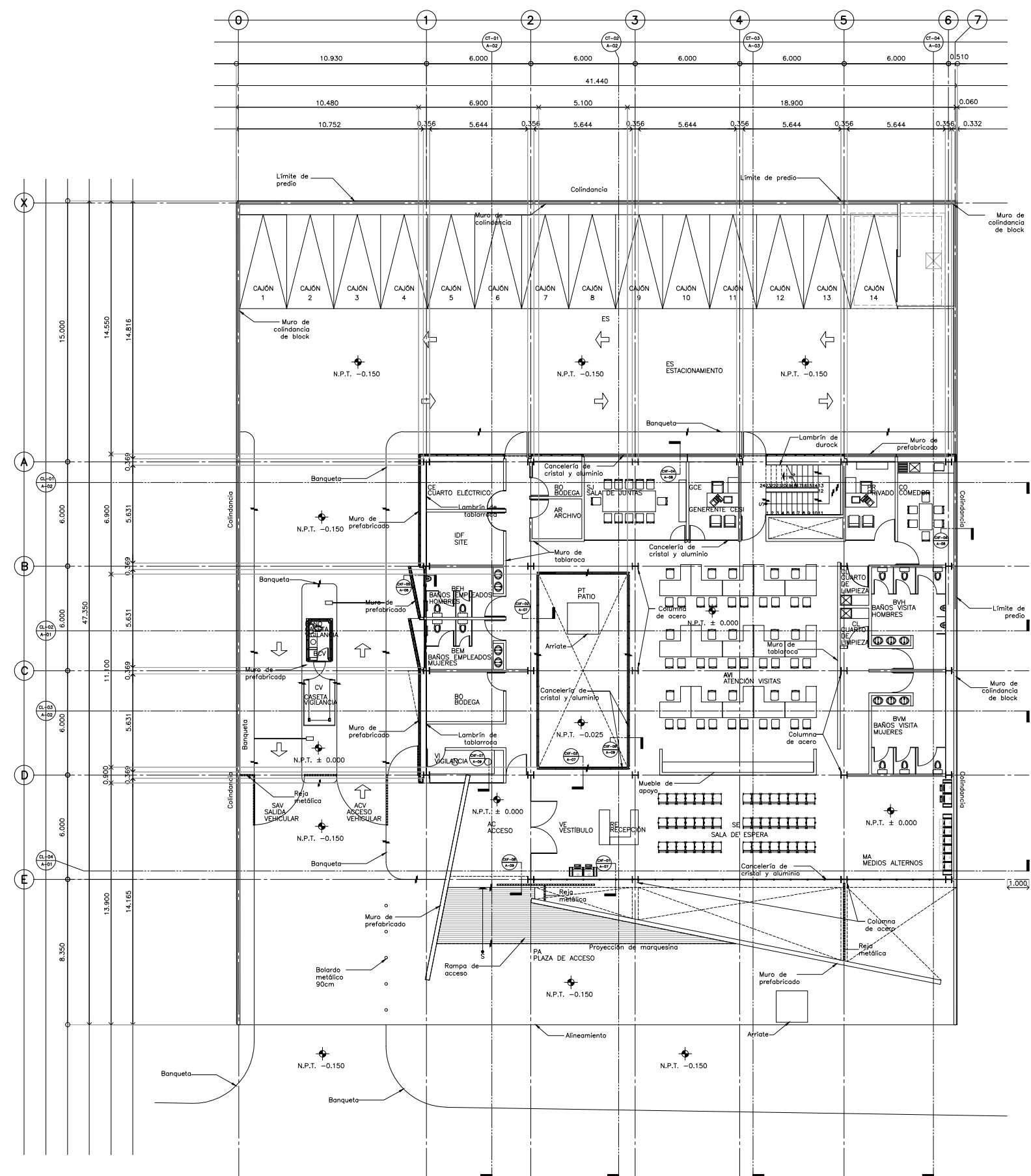
PLANTA ARQUITECTÓNICA NIVEL ±0.00 DETALLE 01
