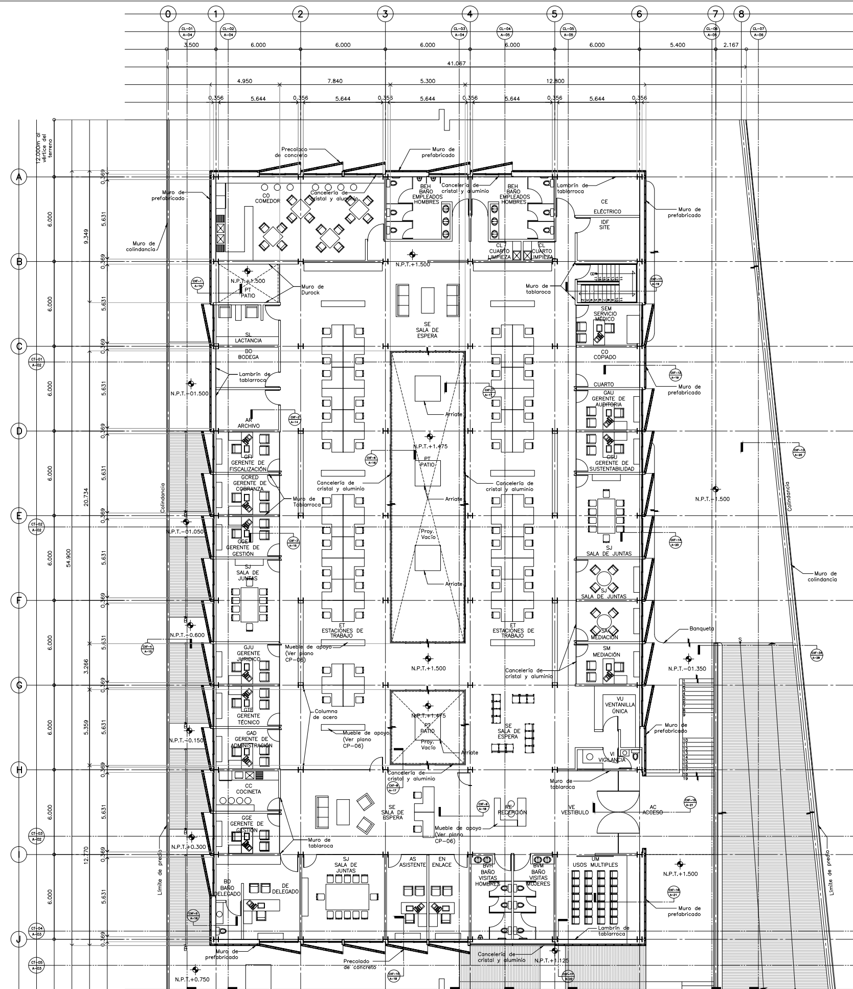
PLANTA ARQUITECTÓNICA NIVEL +1.500 / DETALLE 03
