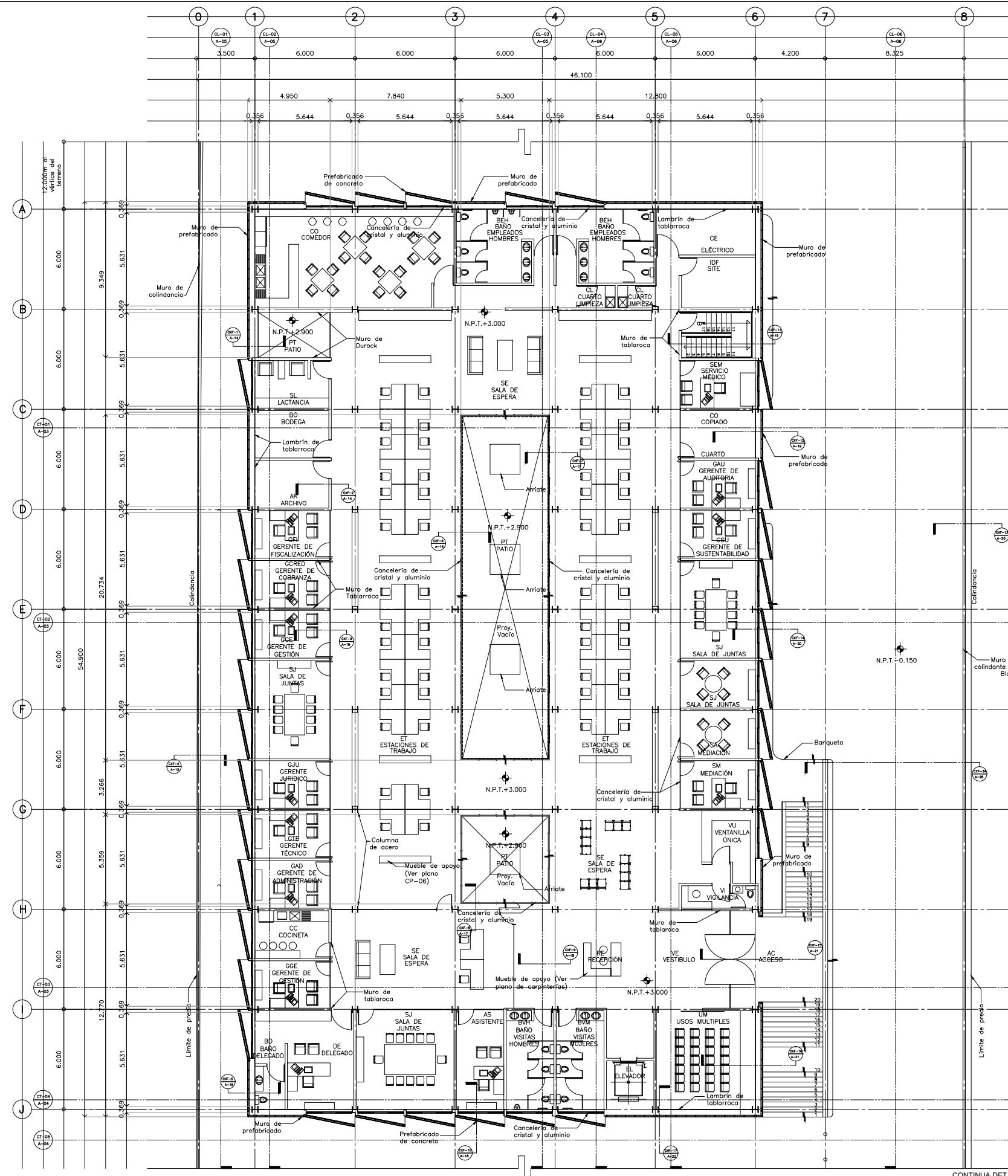
PLANTA ARQUITECTÓNICA NIVEL +3.000 / DETALLE 04
