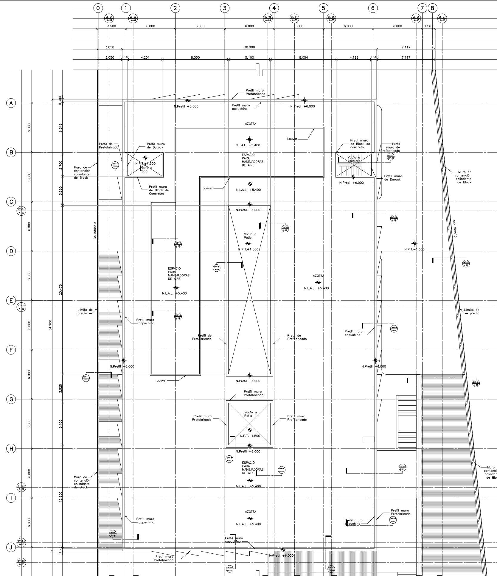
PLANTA ARQUITECTÓNICA NIVEL +5.400 / DETALLE 5
