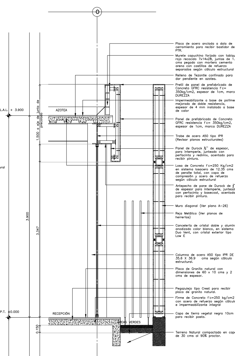
CORTE POR FACHADA CXF-27
