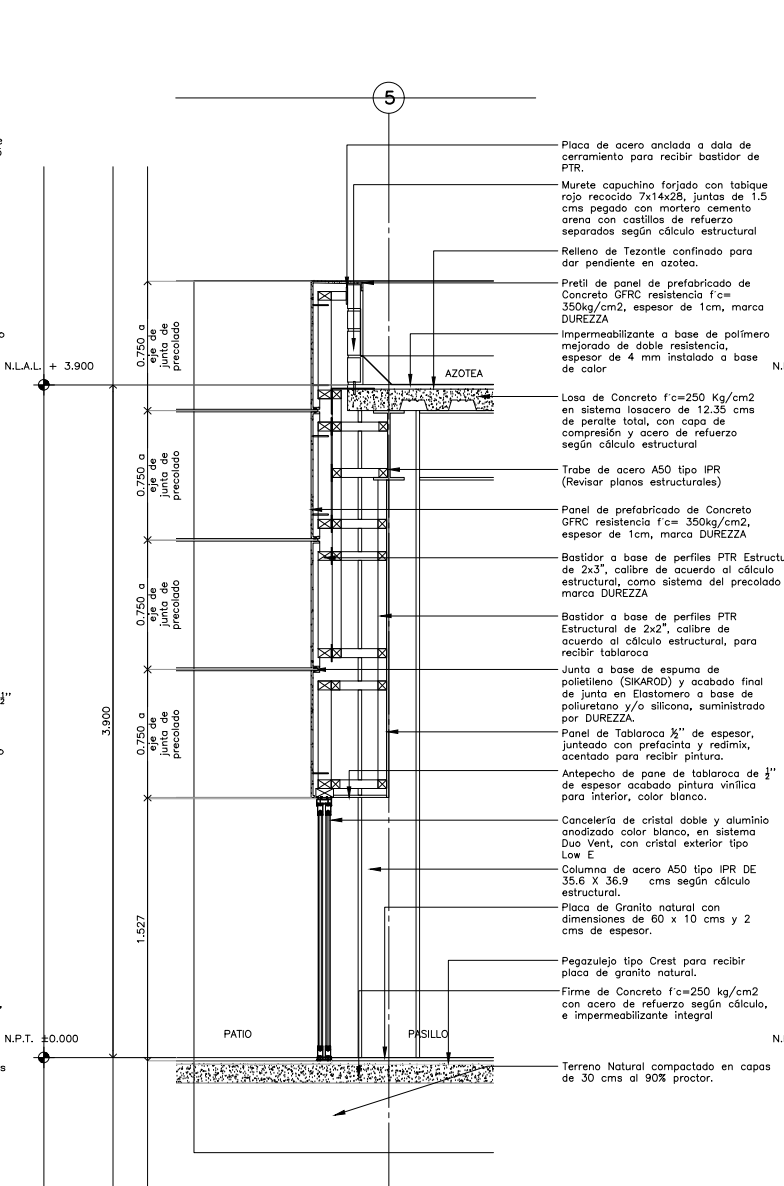
CORTE POR FACHADA CXF-26
