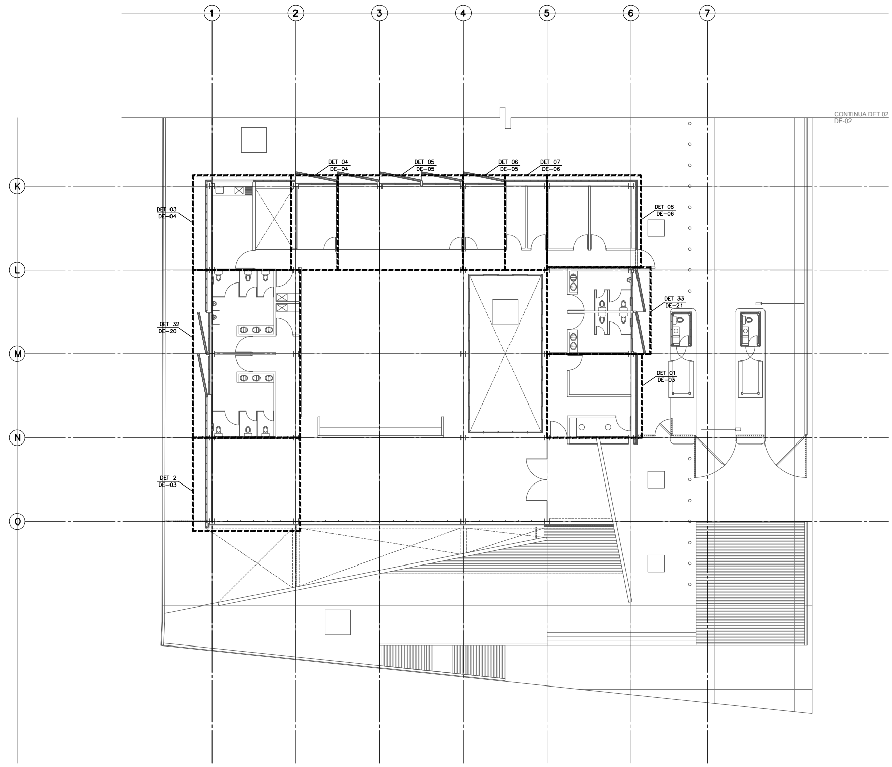
PLANTA ARQUITECTÓNICA PLANO LLAVE DETALLES ESPACIO NIVEL ±0.00
