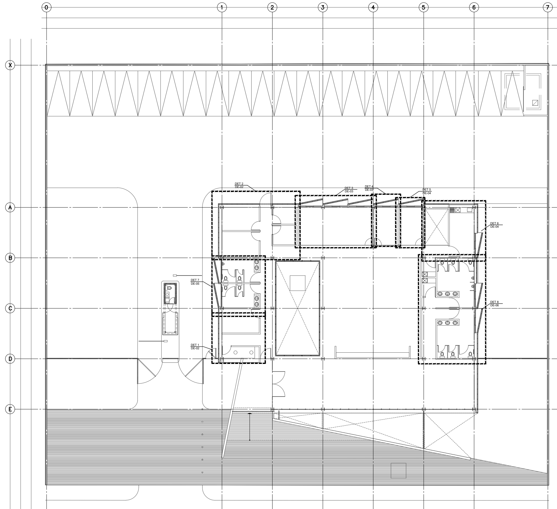
PLANTA ARQUITECTÓNICA N. ±0.000
