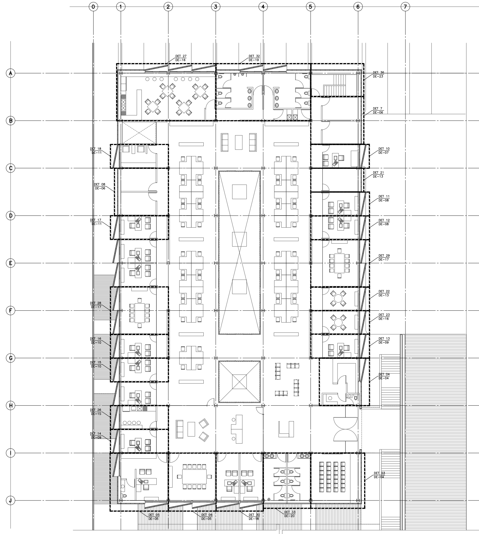
PLANTA ARQUITECTÓNICA NIVEL +3.000 / DETALLE 3
