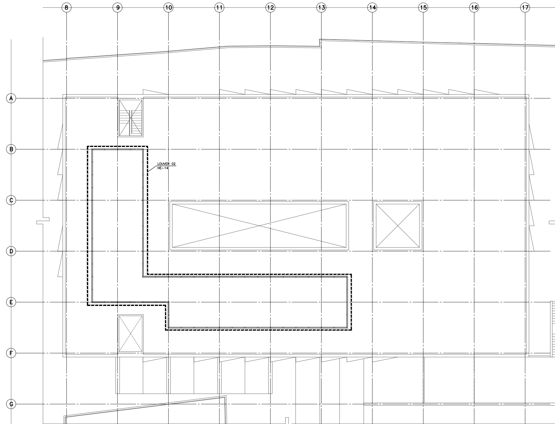
PLANTA ARQUITECTÓNICA HERRERÍAS NIVEL +6.900
