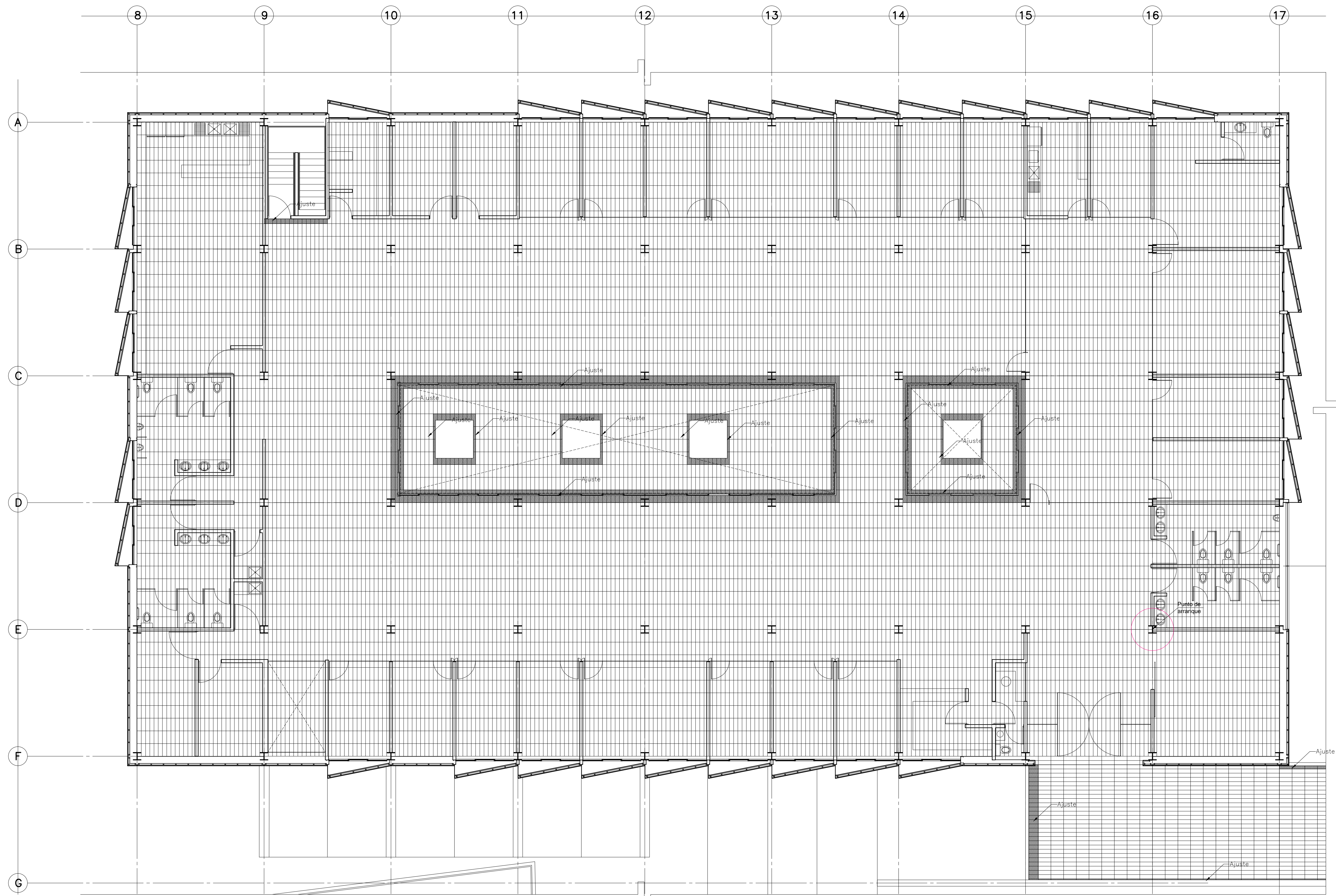
PLANTA ARQUITECTÓNICA DESPIECE DE PISOS NIVEL +3.000
