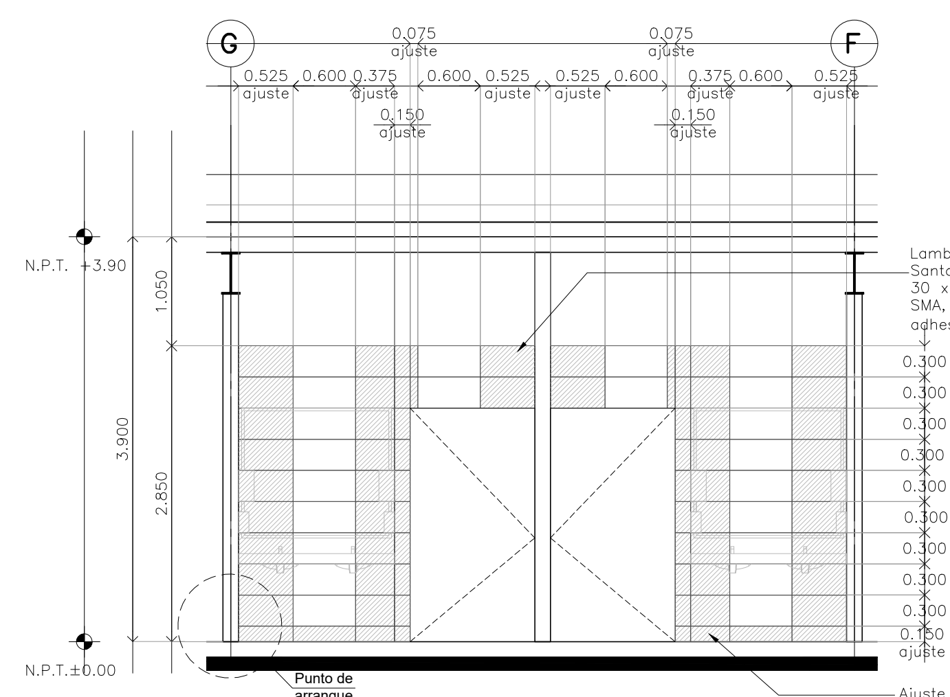
CORTE 05 Detalle 26 Escala: 1:50
