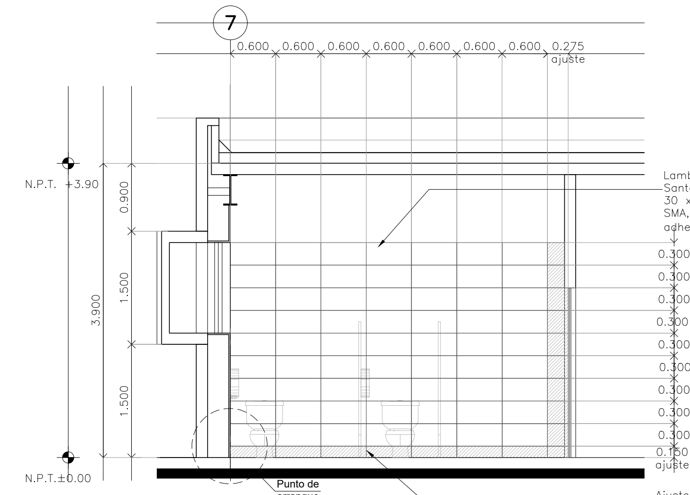
CORTE 02 Detalle 26 Escala: 1:50
