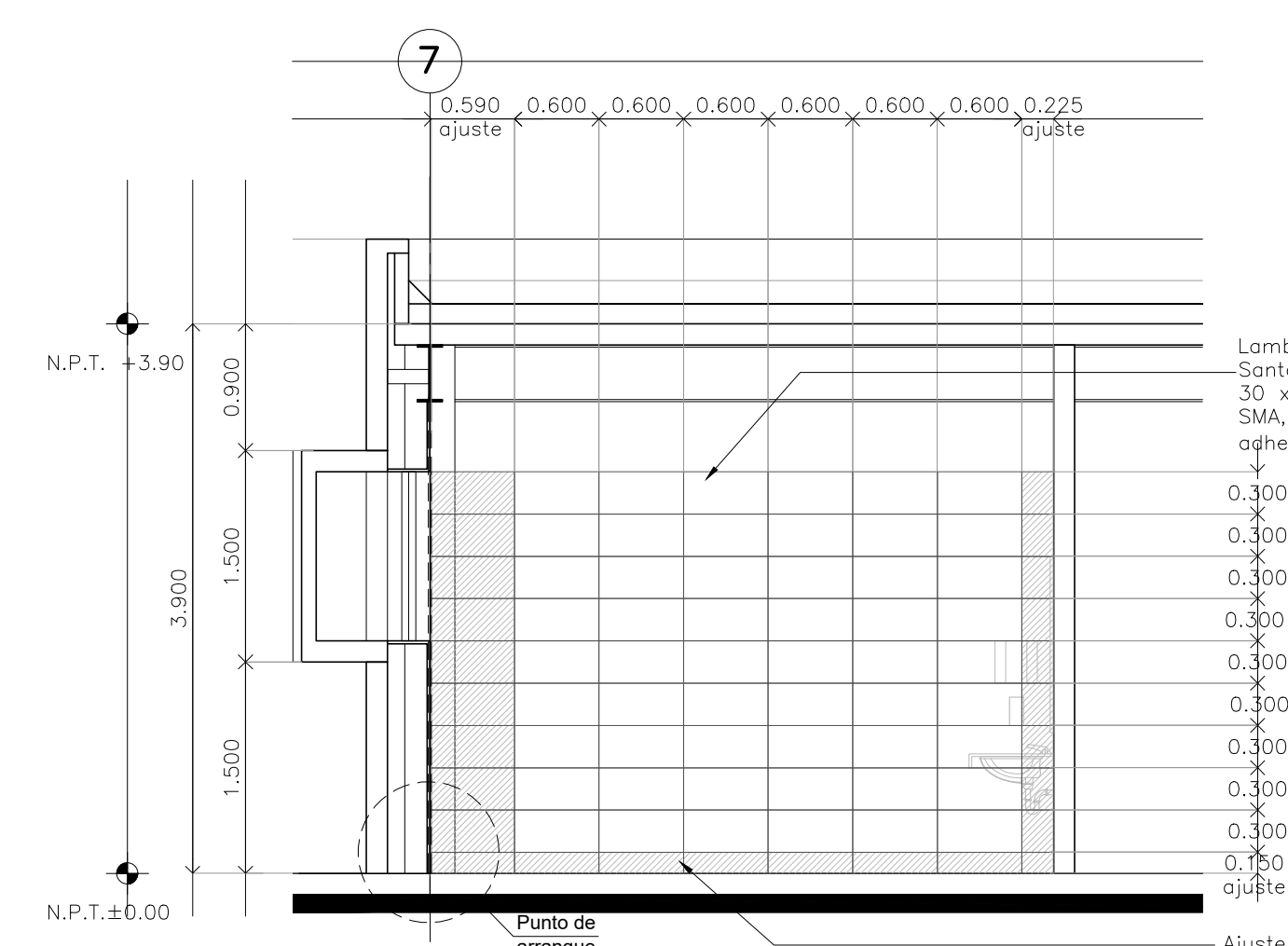
CORTE 04 Detalle 26 Escala: 1:50
