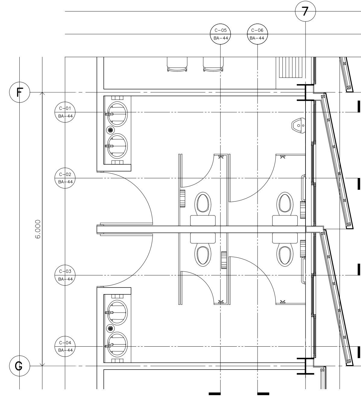
Detalle 26 Planta Sanitarios Visitas / CESI Escala: 1:50
