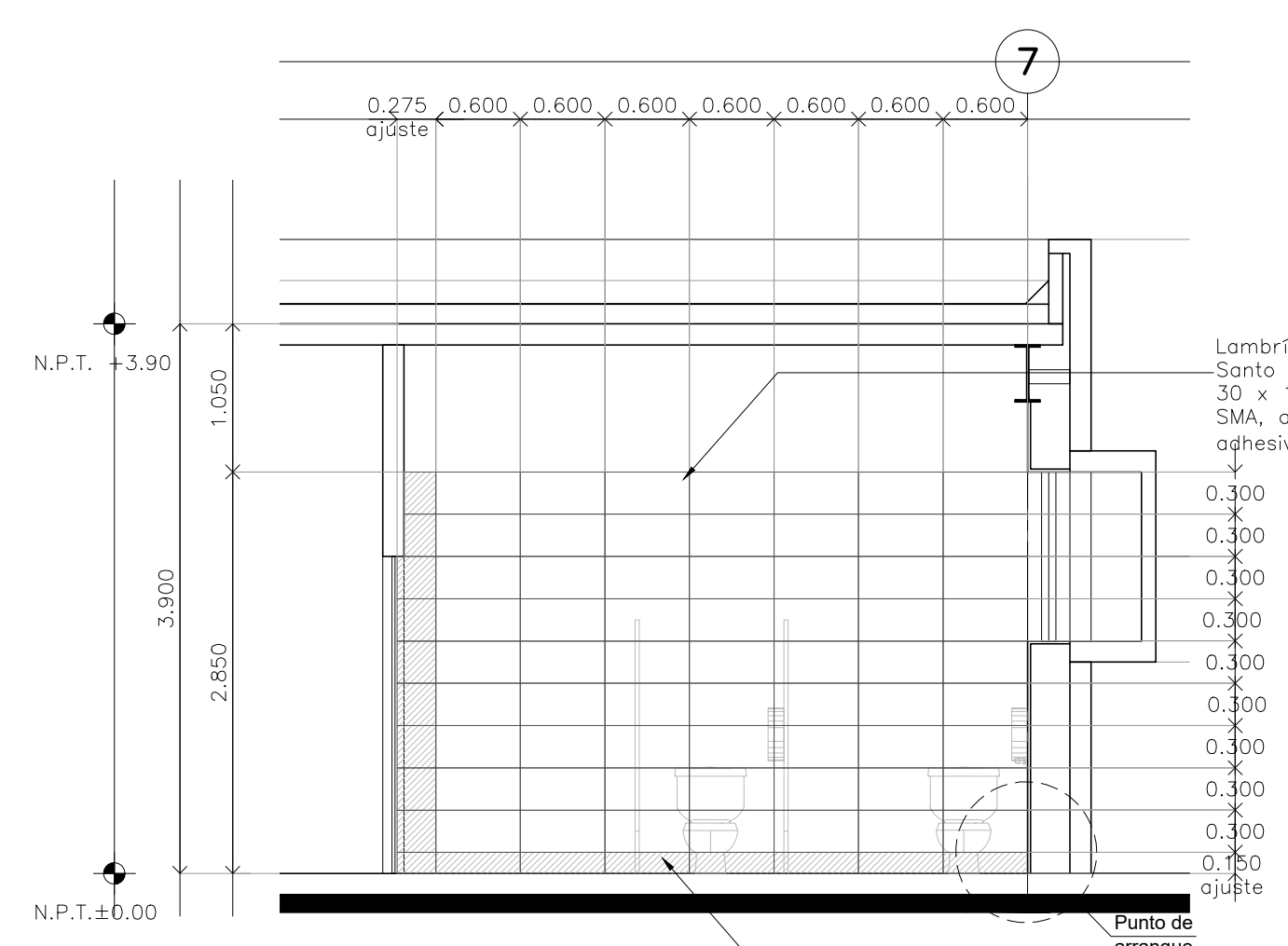
CORTE 03 Detalle 26 Escala: 1:50
