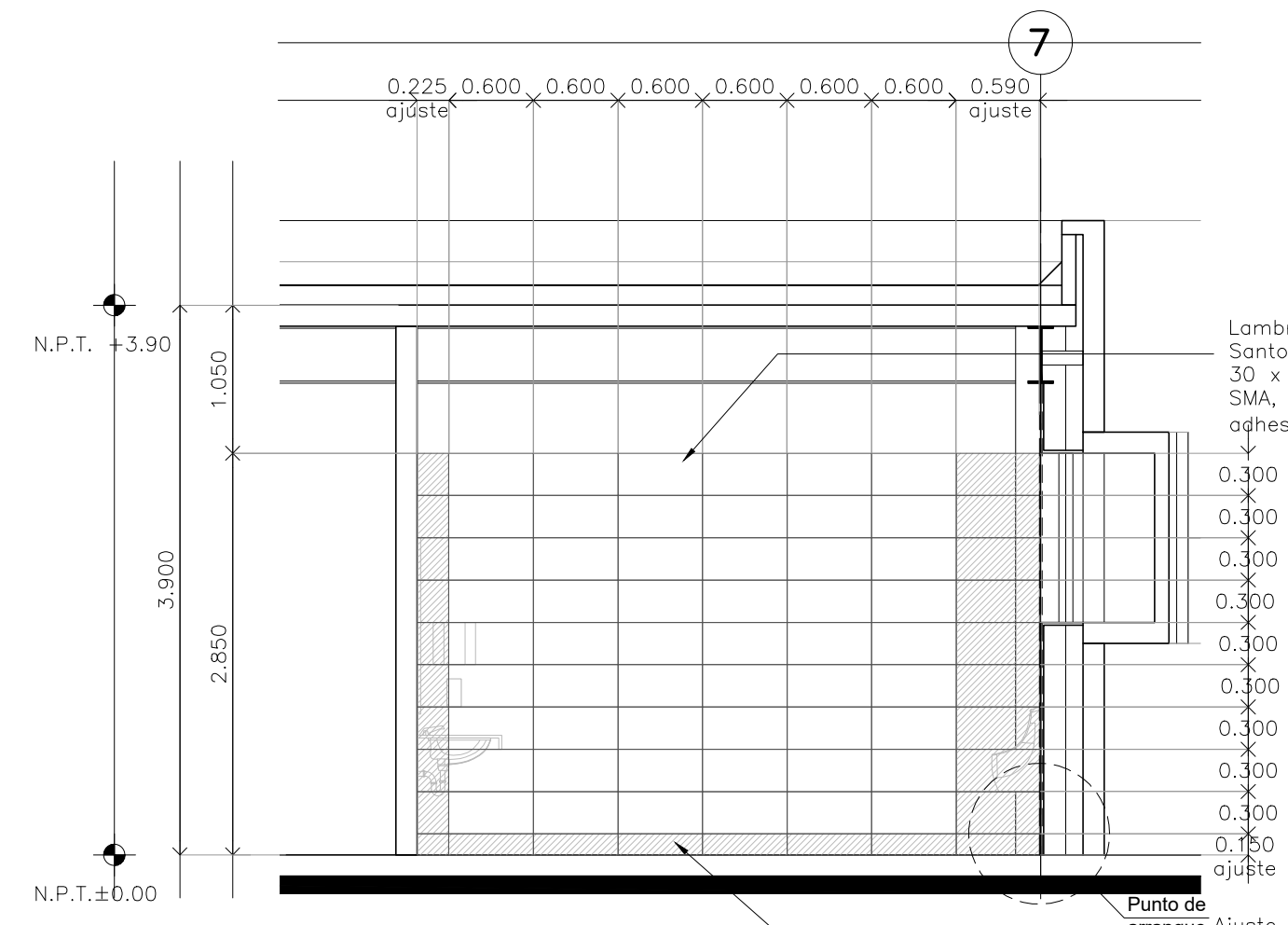
CORTE 01 Detalle 26 Escala: 1:50
