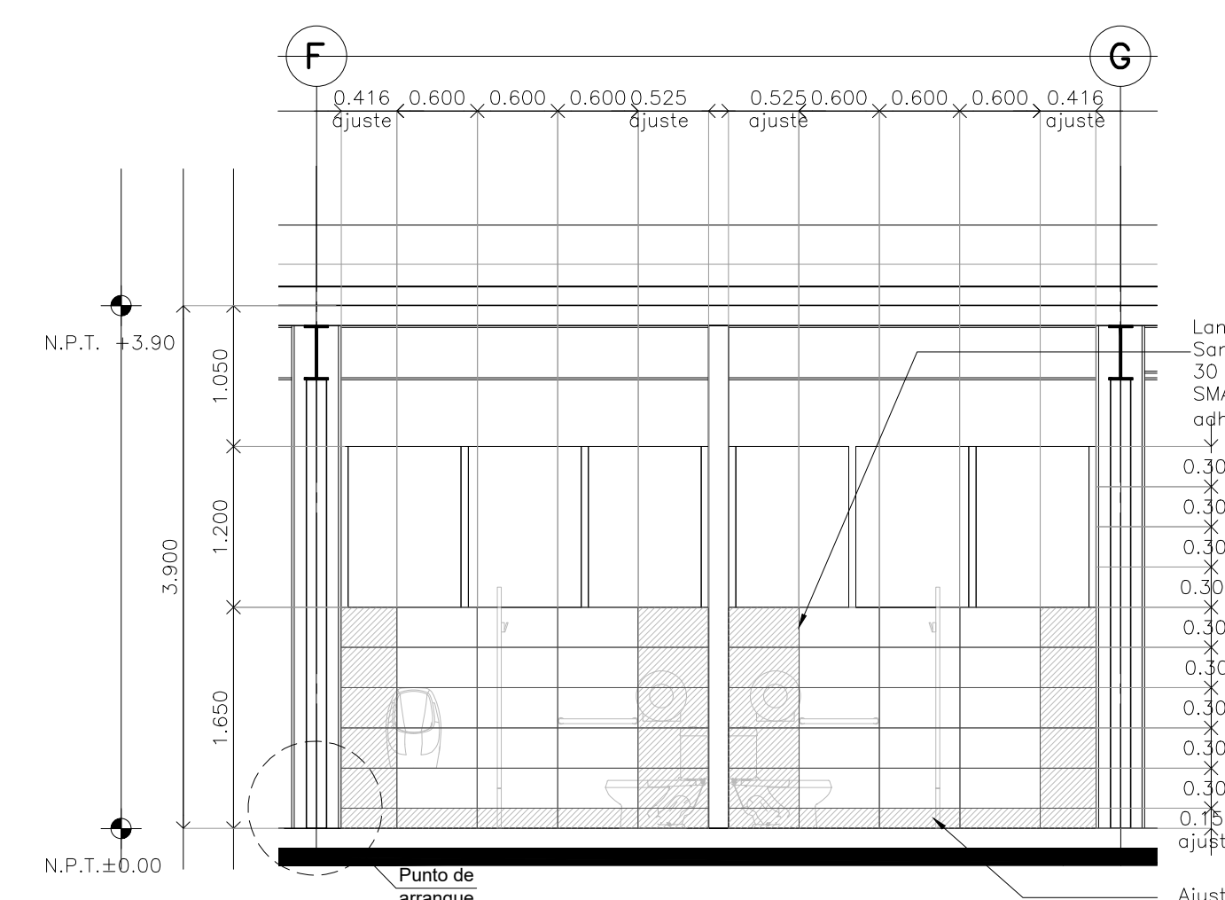
CORTE 06 Detalle 26 Escala: 1:50
