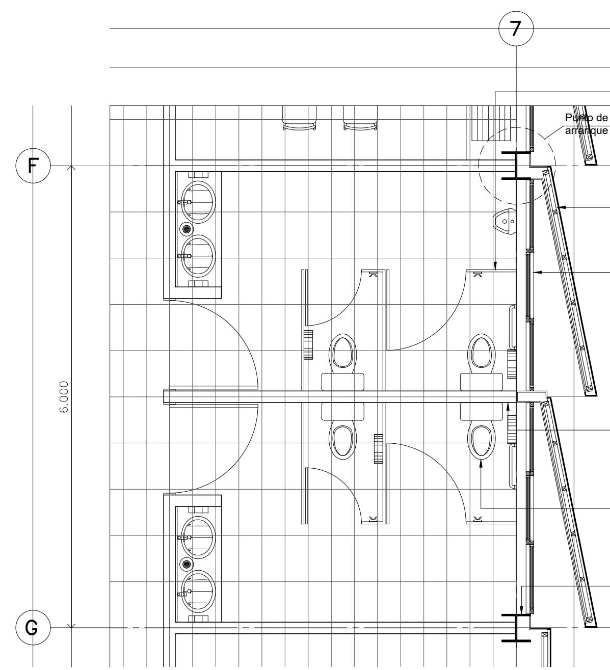
Detalle 26 Despiece de pisos Planta Sanitarios Visitas / CESI Escala: 1:50
