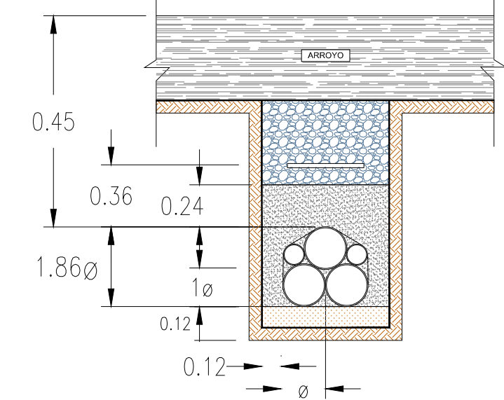
CORTE A-A BANCO DE DUCTOS SUBTERRANEO ESC: S/E
