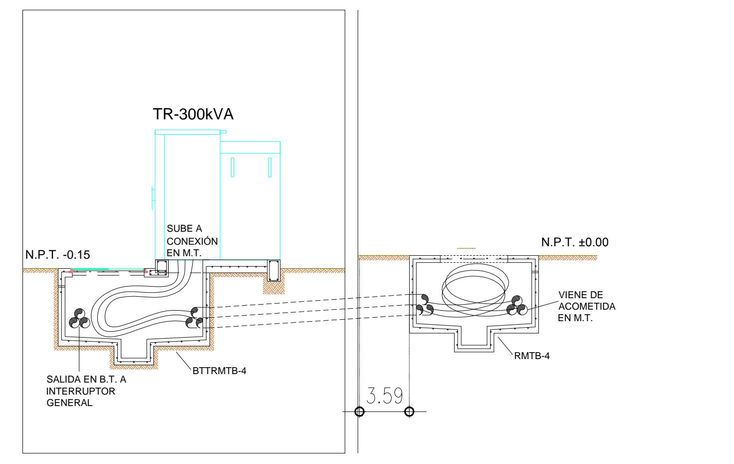
CORTE B-B REGISTROS M.T. ESC: S/E
