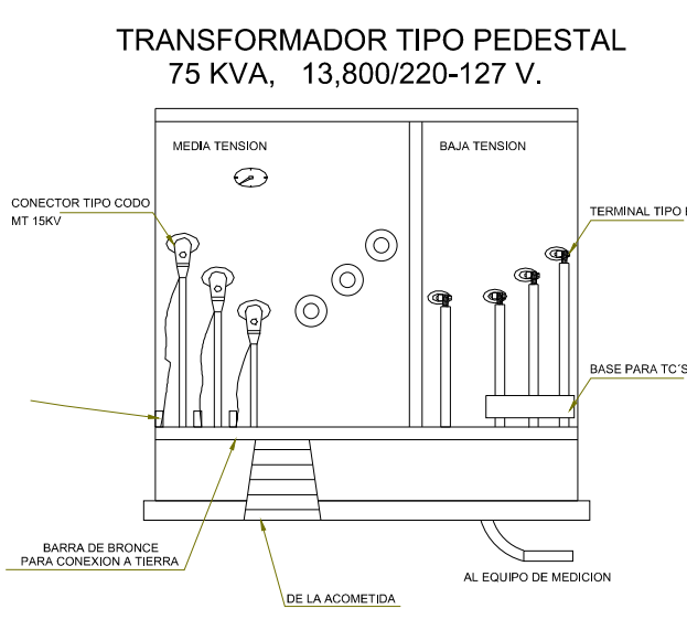
DETALLE TIPO CONEXIÓN DE TRANSFORMADOR ESC: S/E
