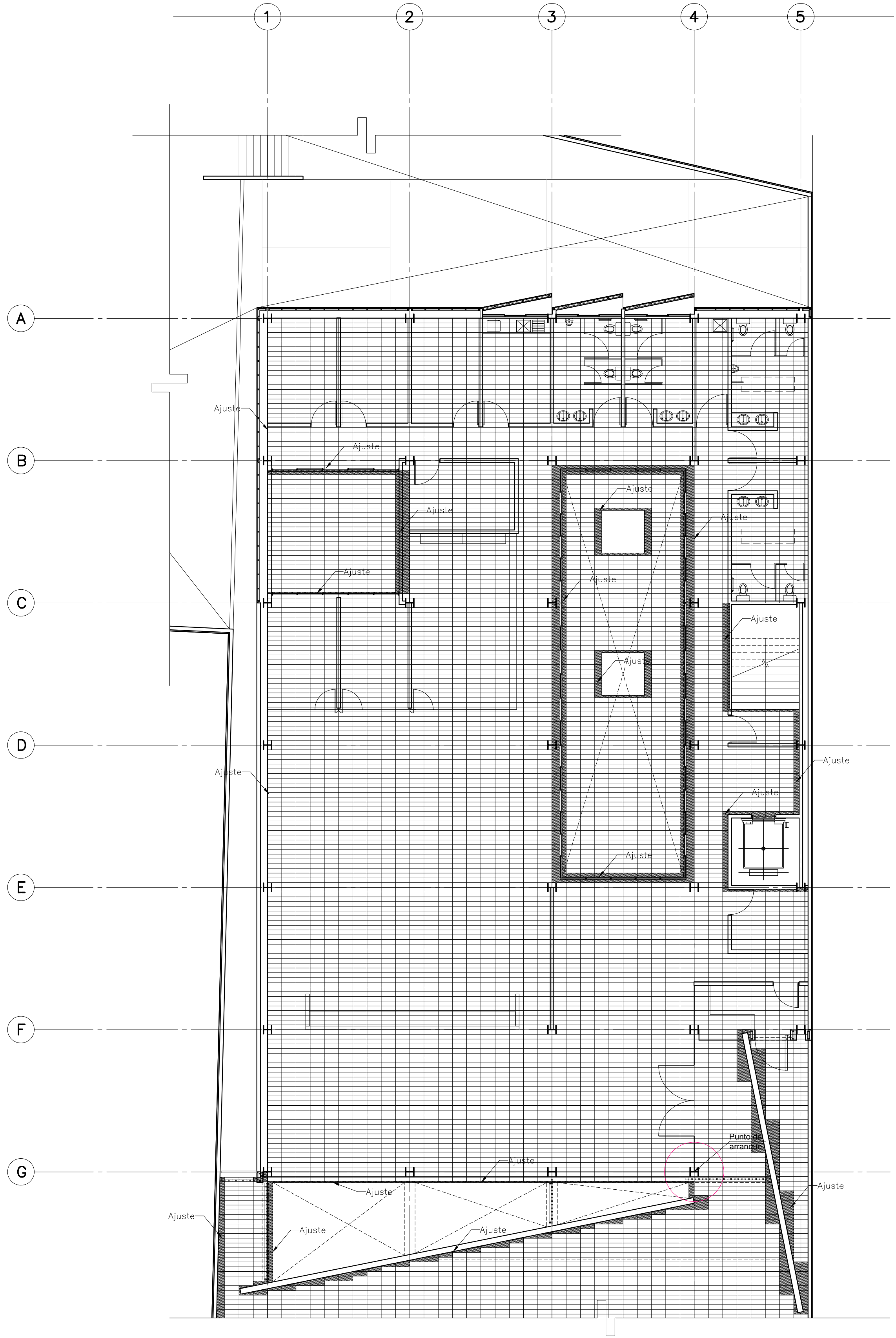
PLANTA DE DESPIECES NIVEL +1.500
