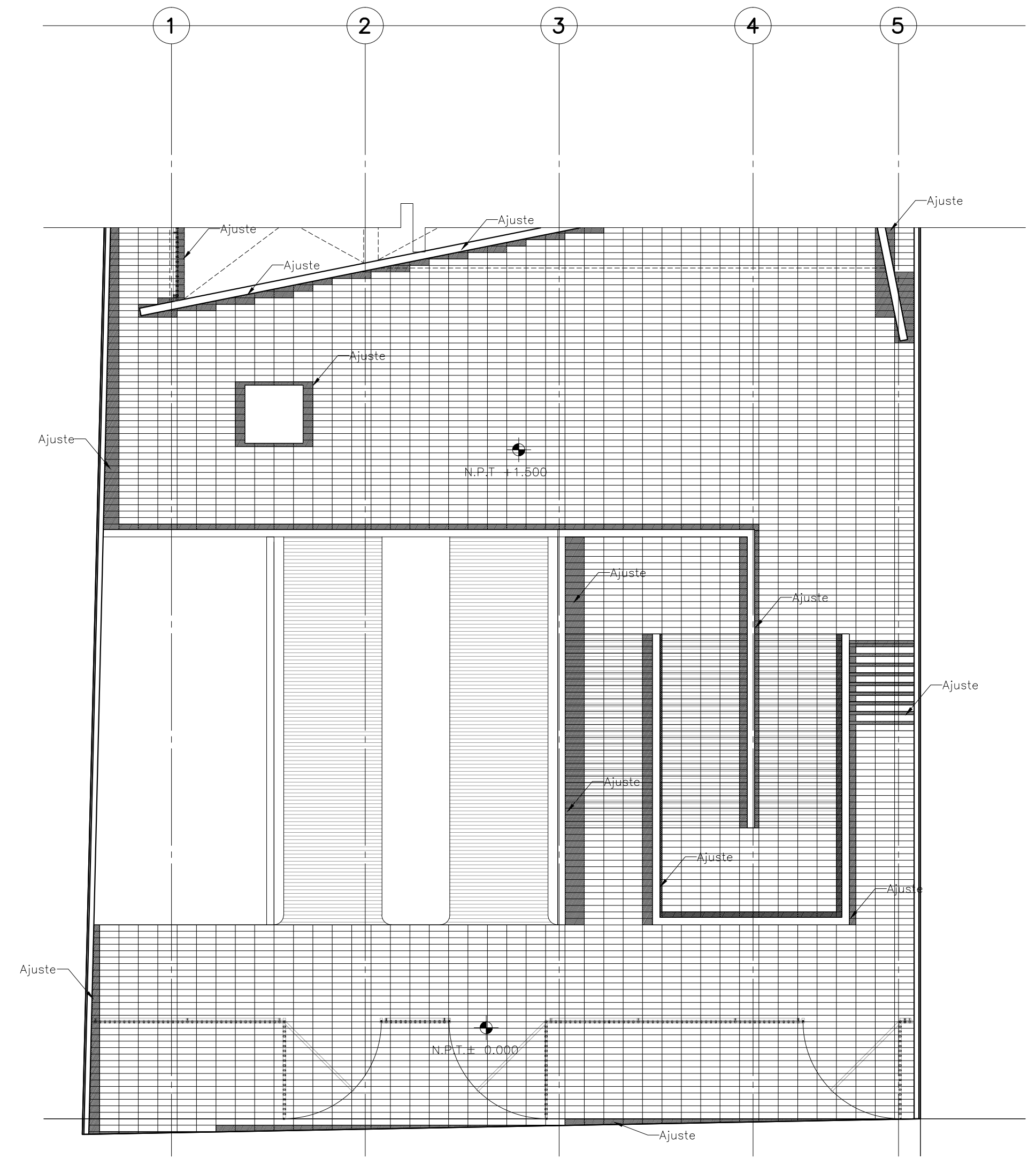
PLANTA DE DESPIECES NIVELES ±0.000 Y +1.500
