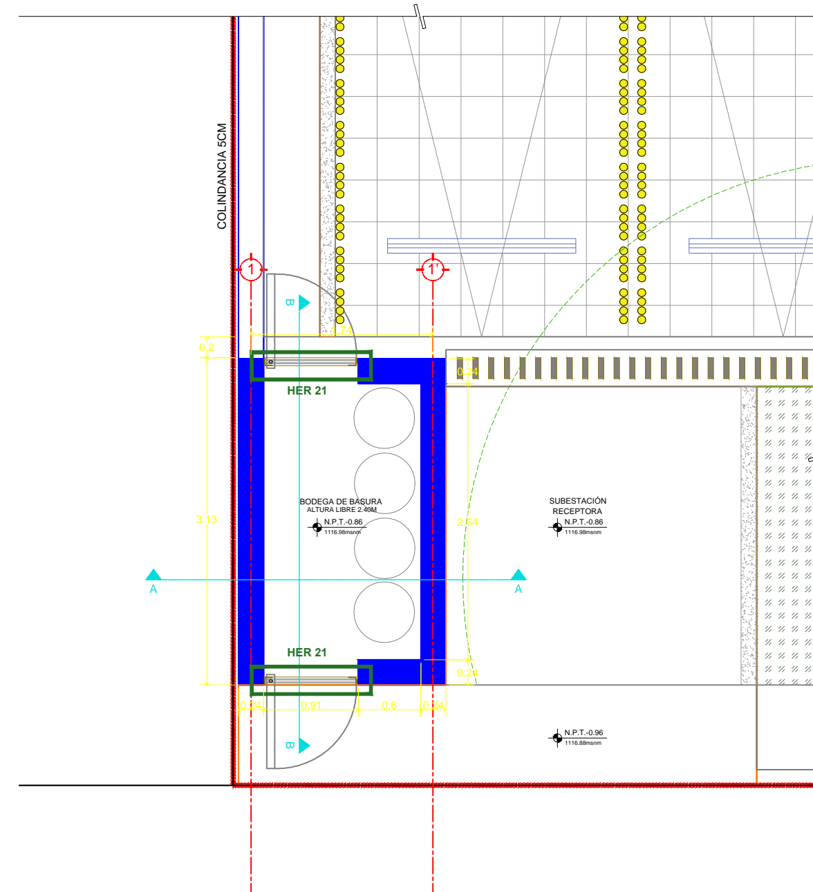
2 PLANTA BAJA ESC 1:50
