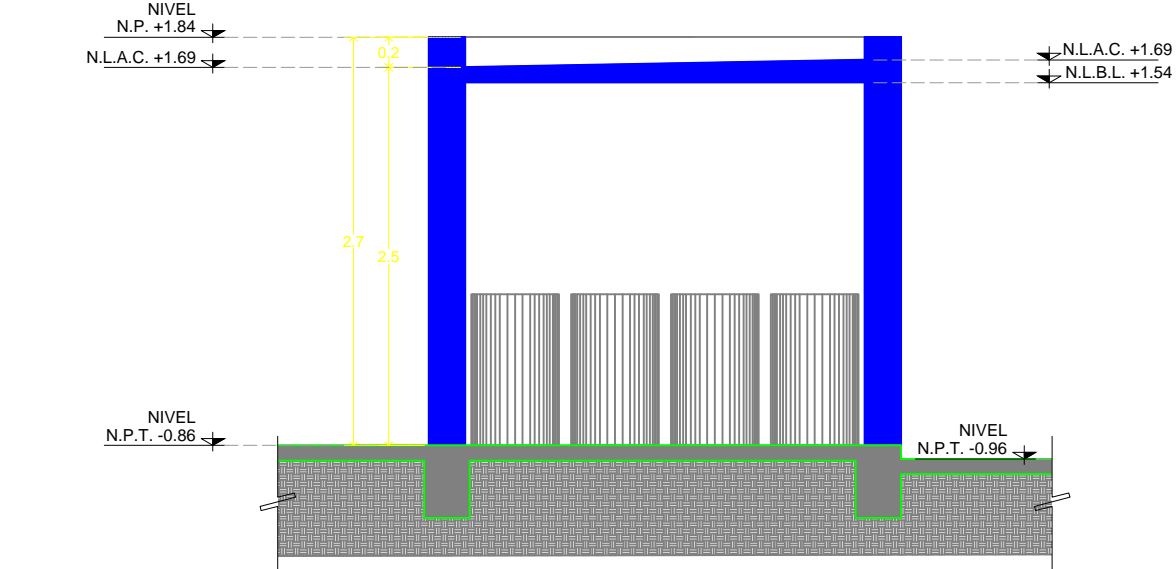
6 CORTE LONGITUDINAL B-B ESC 1:50
