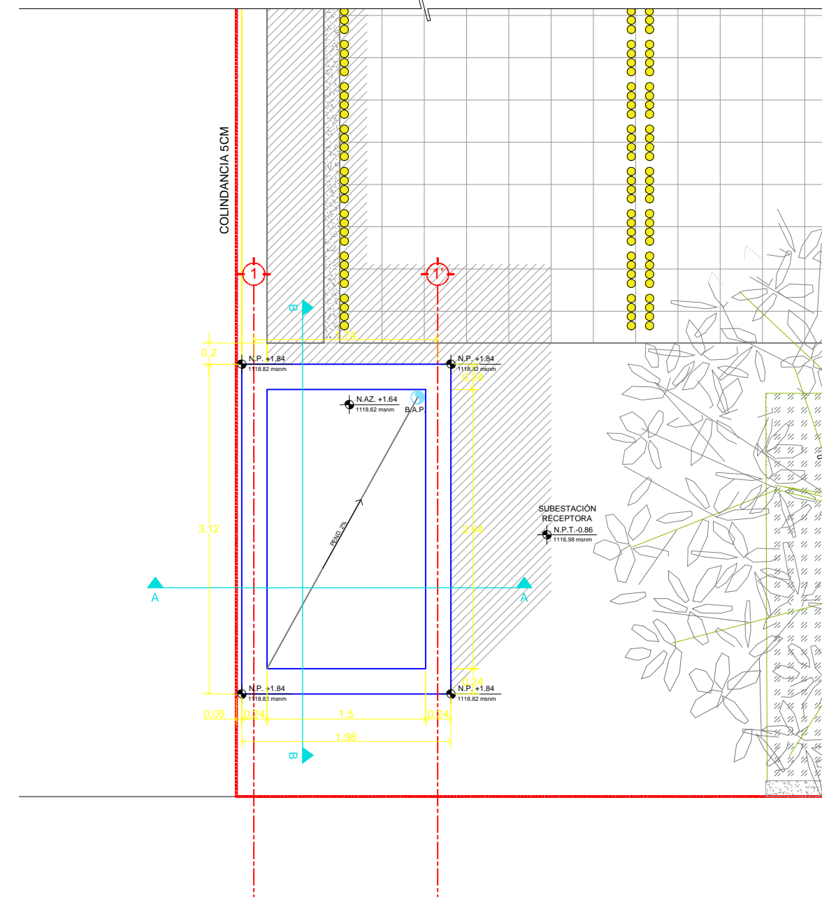
1 PLANTA AZOTEA ESC 1:50
