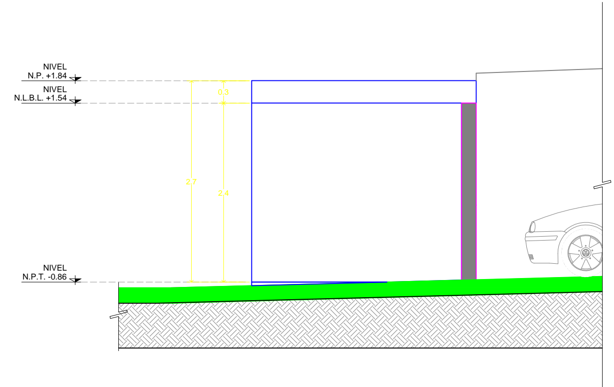
4 ALZADO LATERAL ESC 1:50
