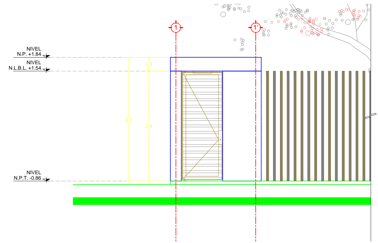
3 ALZADO FRONTAL ESC 1:50
