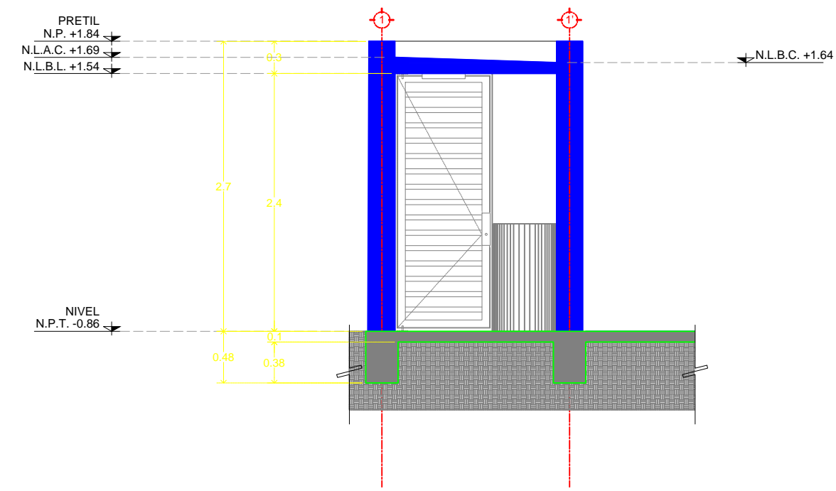
5 CORTE TRANSVERSAL A-A ESC 1:50
