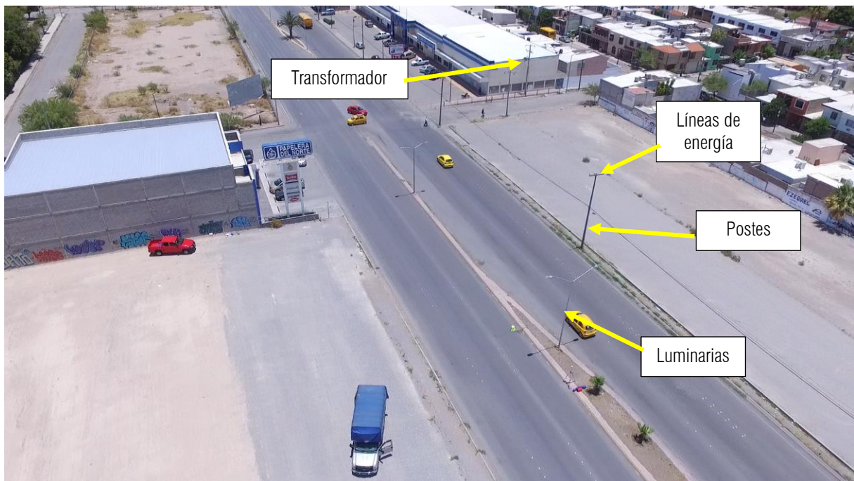
Figura 4.32 Infraestructura de CFE.
