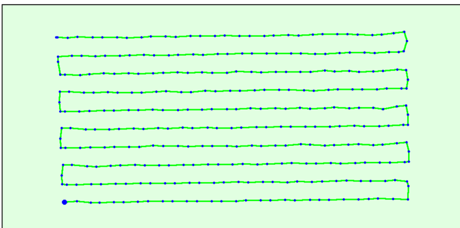
Figura 4.1 Vista superior de la posición inicial de cada imagen. La línea verde sigue el recorrido del dron y el punto azul grande la posición de las imágenes.
