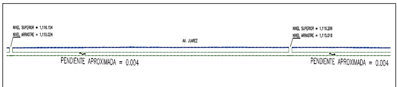
Figura 4.30 Perfil estimado de los pozos de visita.
