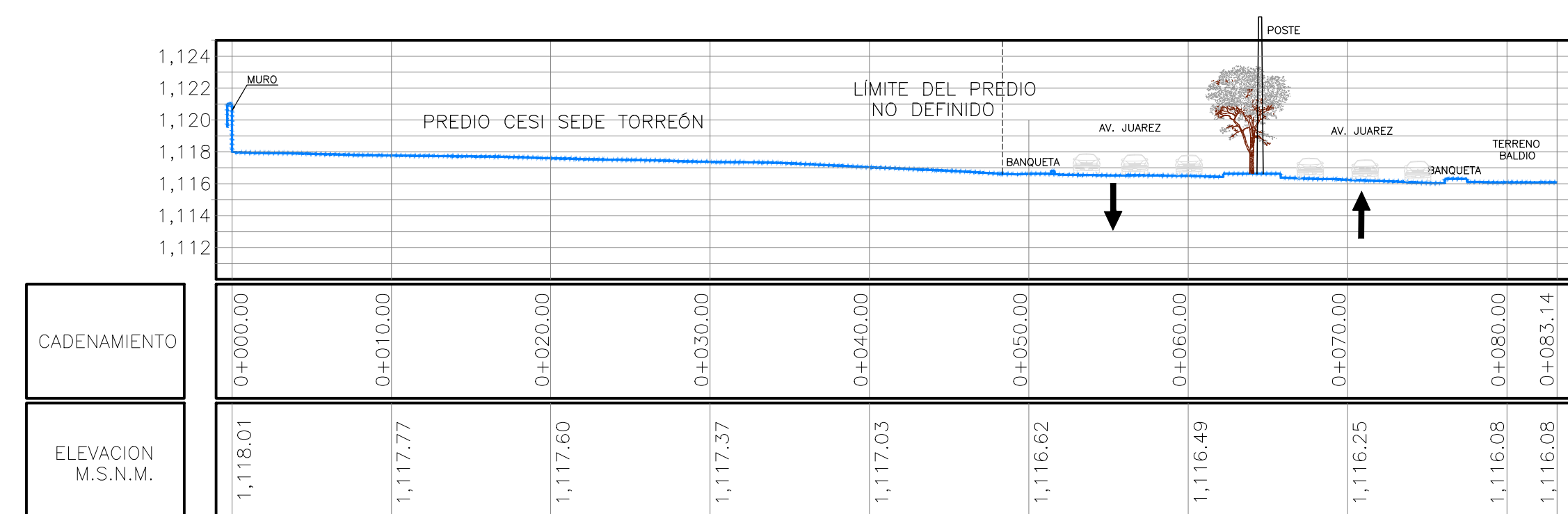
PERFIL 2 ESCALA HORIZONTAL 1 : 100 ESCALA VERTICAL 1 : 100
