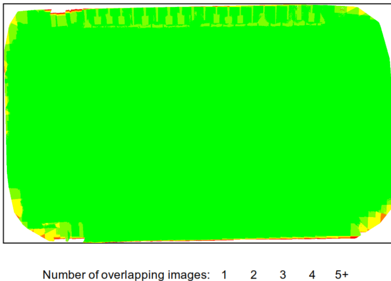
Figura 4.3 Número de imágenes superpuestas calculadas para cada píxel del Ortomosaico. Las áreas rojas y amarillas indican un traslape bajo. Las áreas verdes indican un traslape alto, para el cual se genera resultados confiables.
