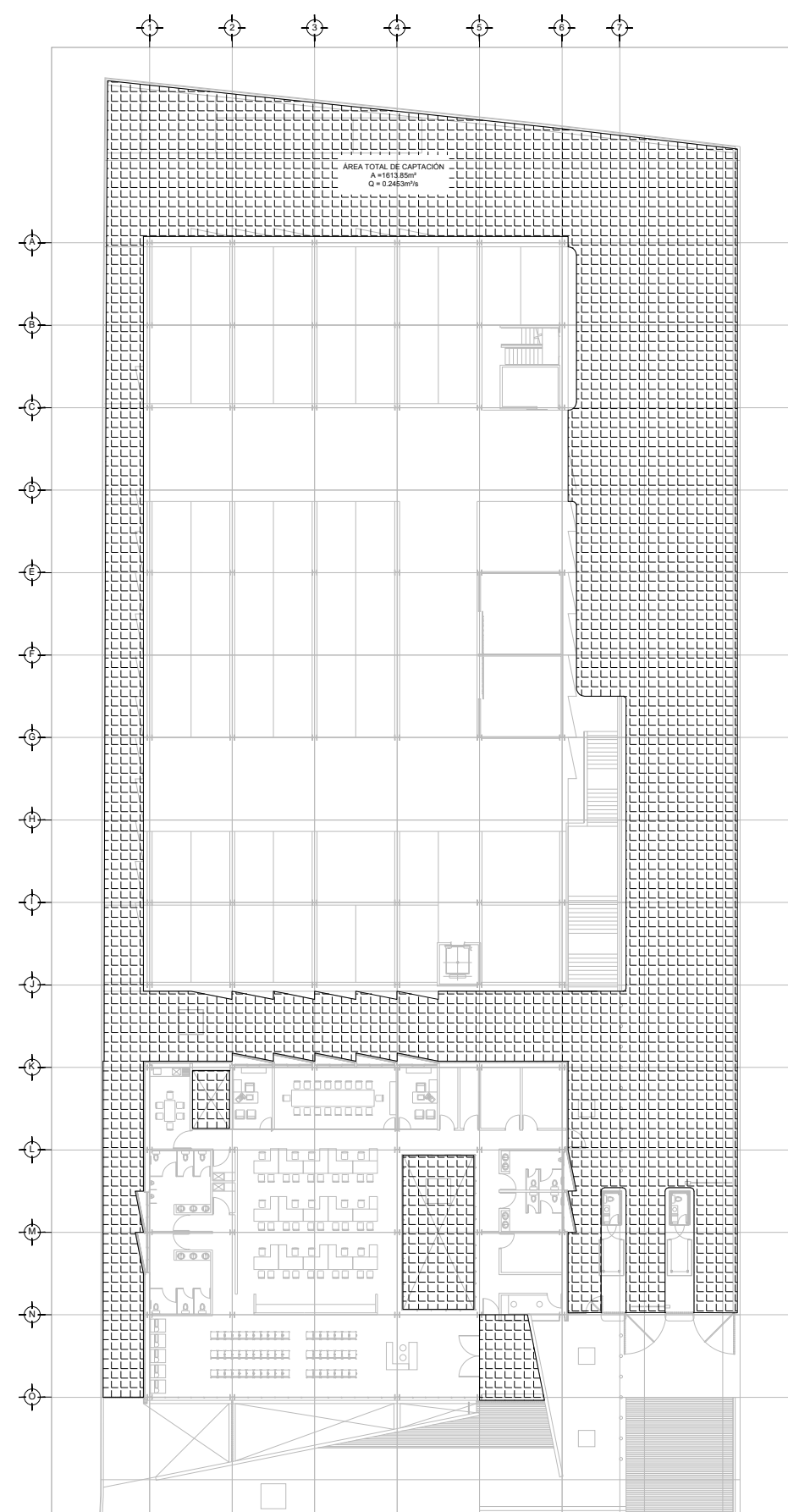
DRENAJE PLUVIAL - PLANO LLAVE PLANTA - ESTACIONAMIENTO - NIVELES ±0.00/ -0.15 ESC. 1:200
