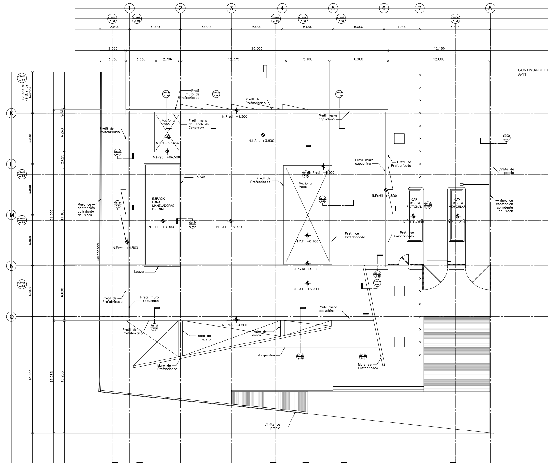
PLANTA ARQUITECTÓNICA NIVEL +3.900 / DETALLE 05
