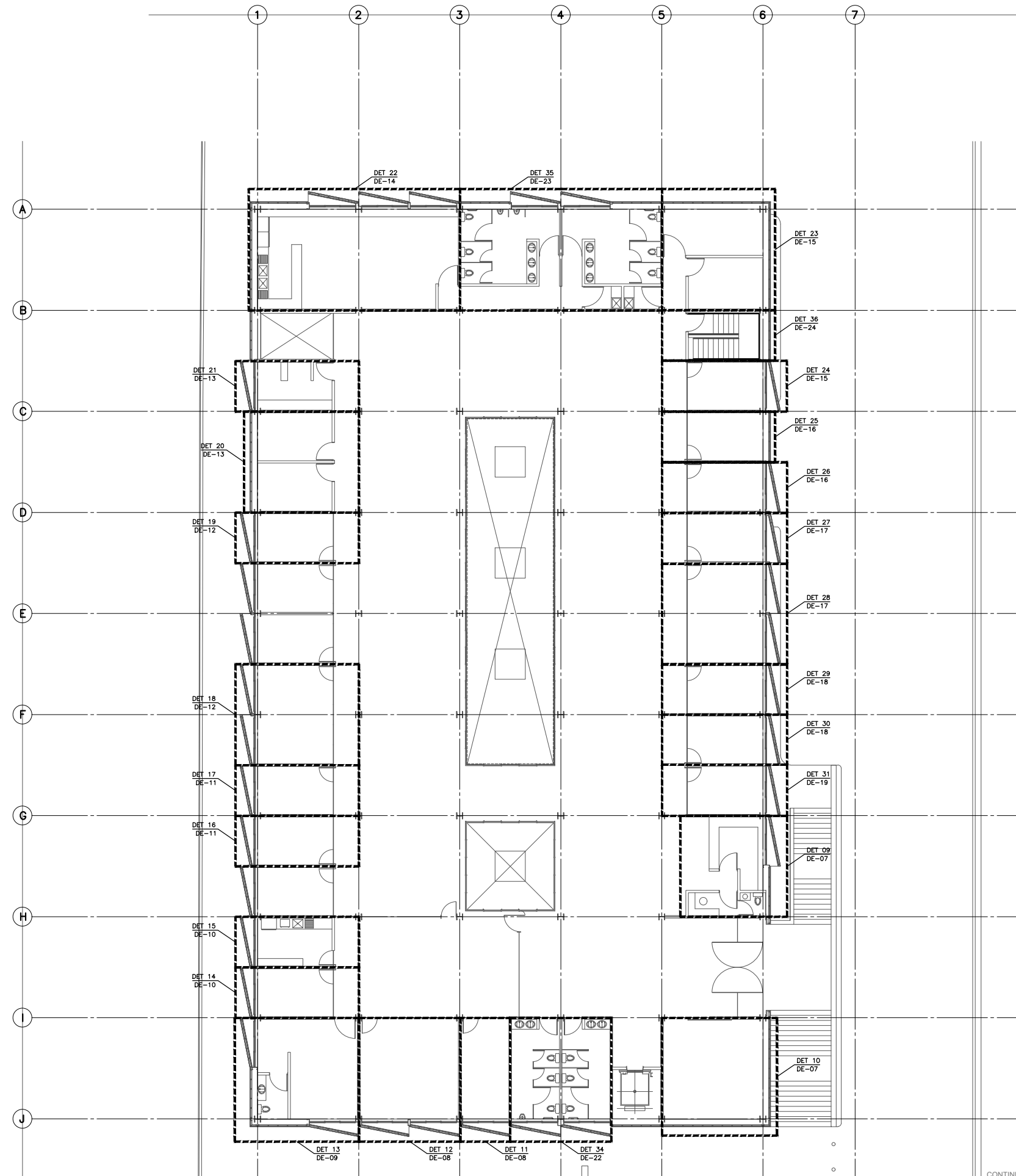
PLANTA ARQUITECTÓNICA PLANO LLAVE DETALLES ESPACIO NIVEL +3.000
