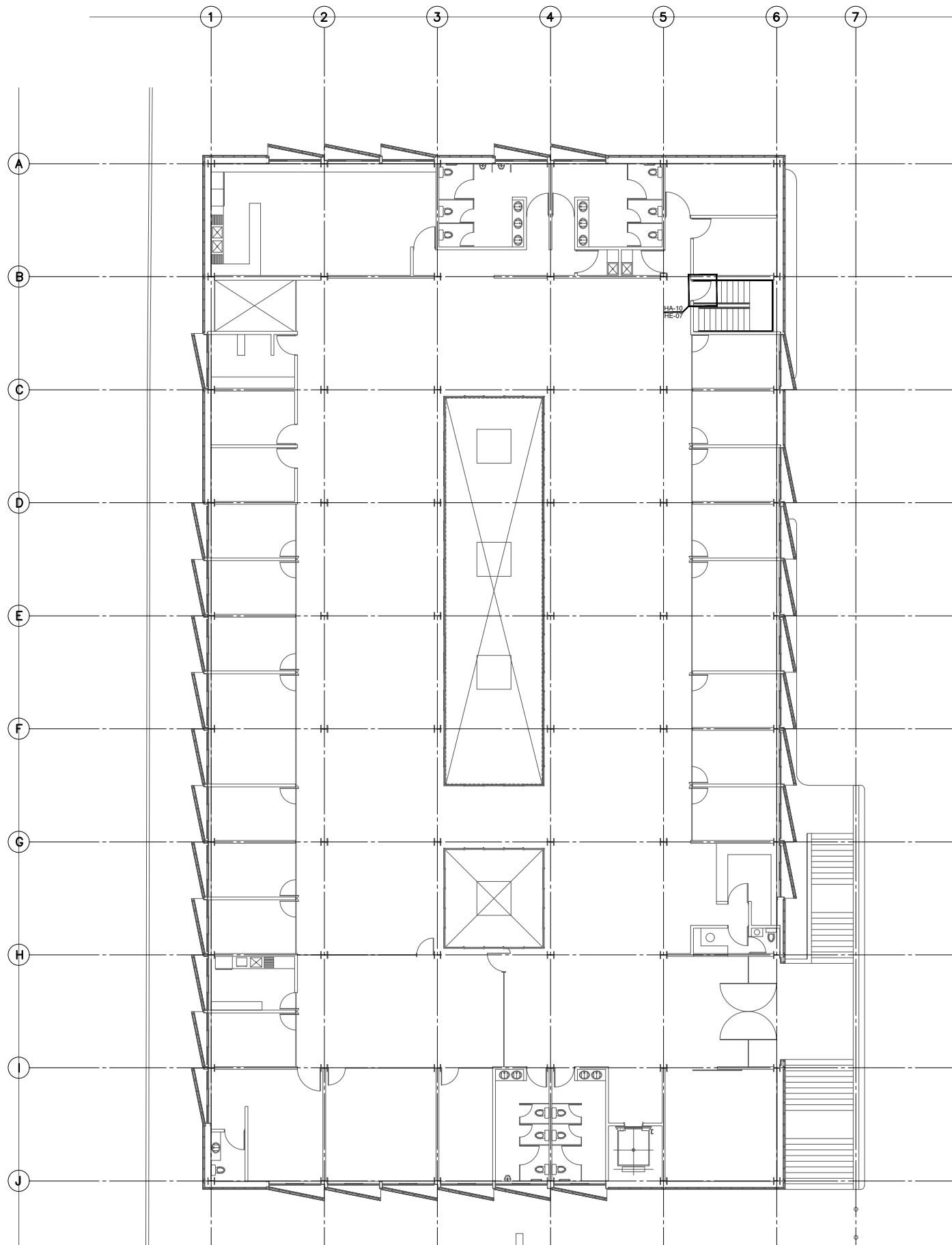
PLANTA ARQUITECTÓNICA PLANO LLAVE HERRERÍAS NIVEL +3.000
