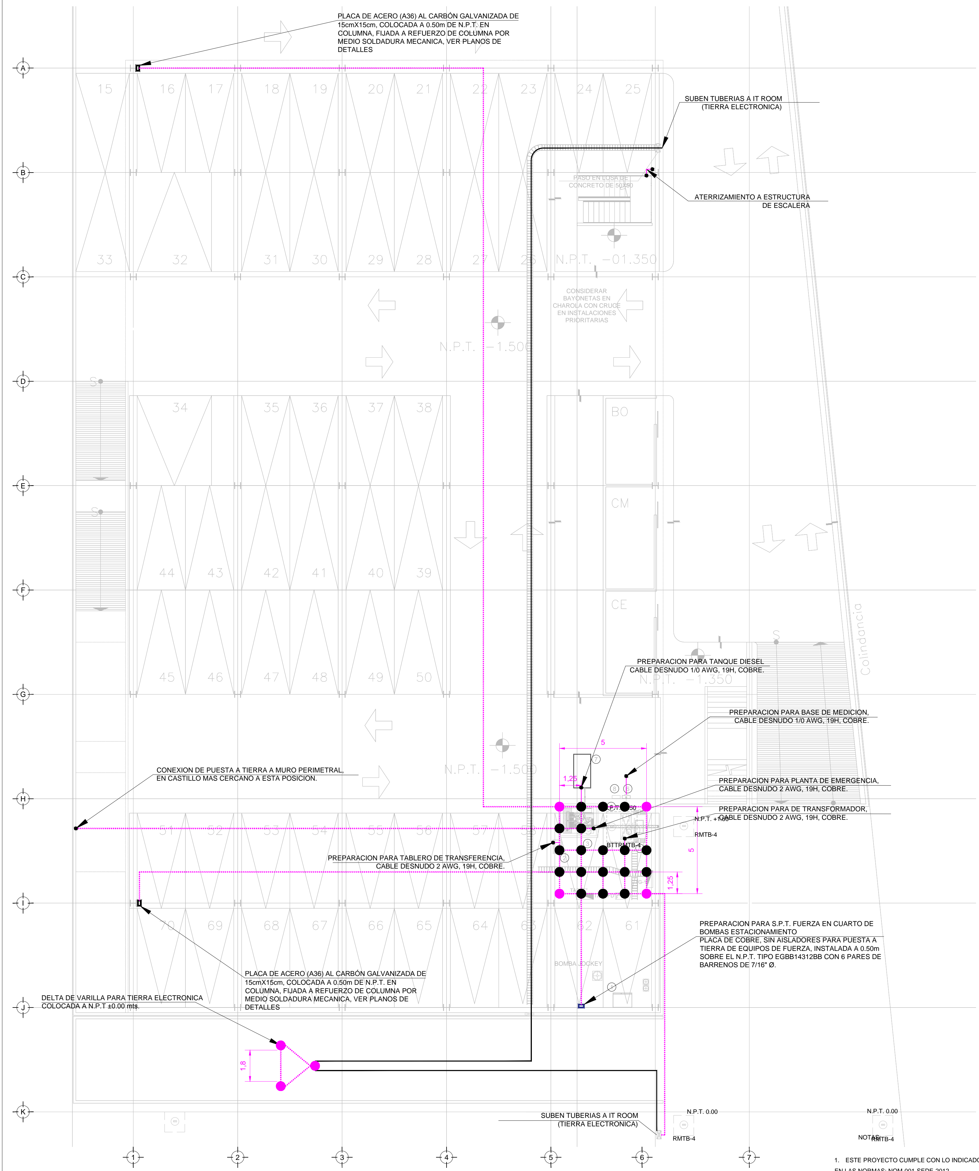
TENDIDO DE INSTALACION ELÉCTRICA (SPT MALLA) N.P.T. -1.50mts. ESC: 1:125
