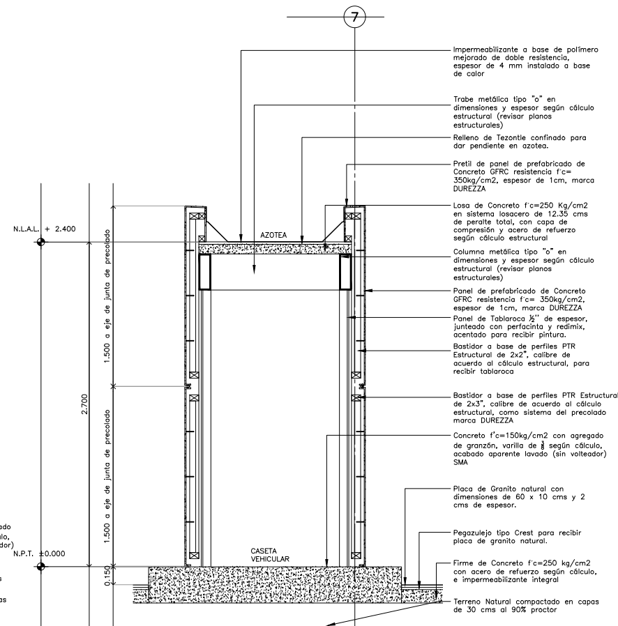
CORTE POR FACHADA CFX-33
