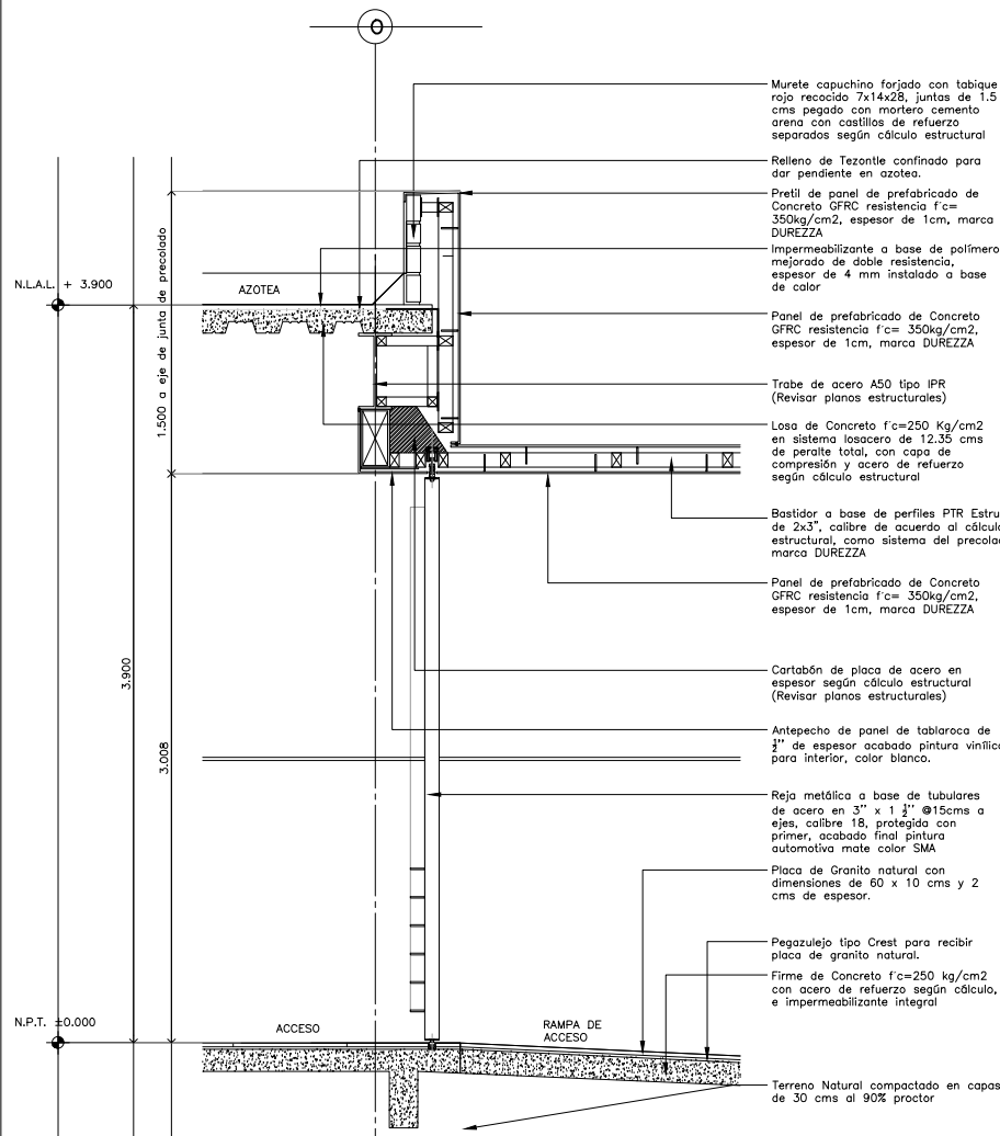
CORTE POR FACHADA CFX-31
