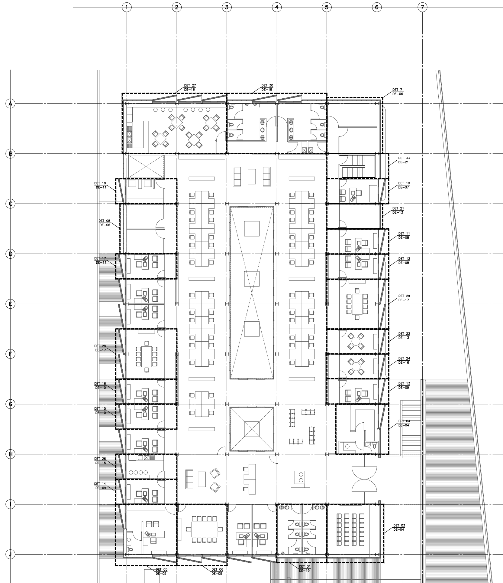
PLANTA ARQUITECTÓNICA NIVEL +1.50 / DETALLE 3
