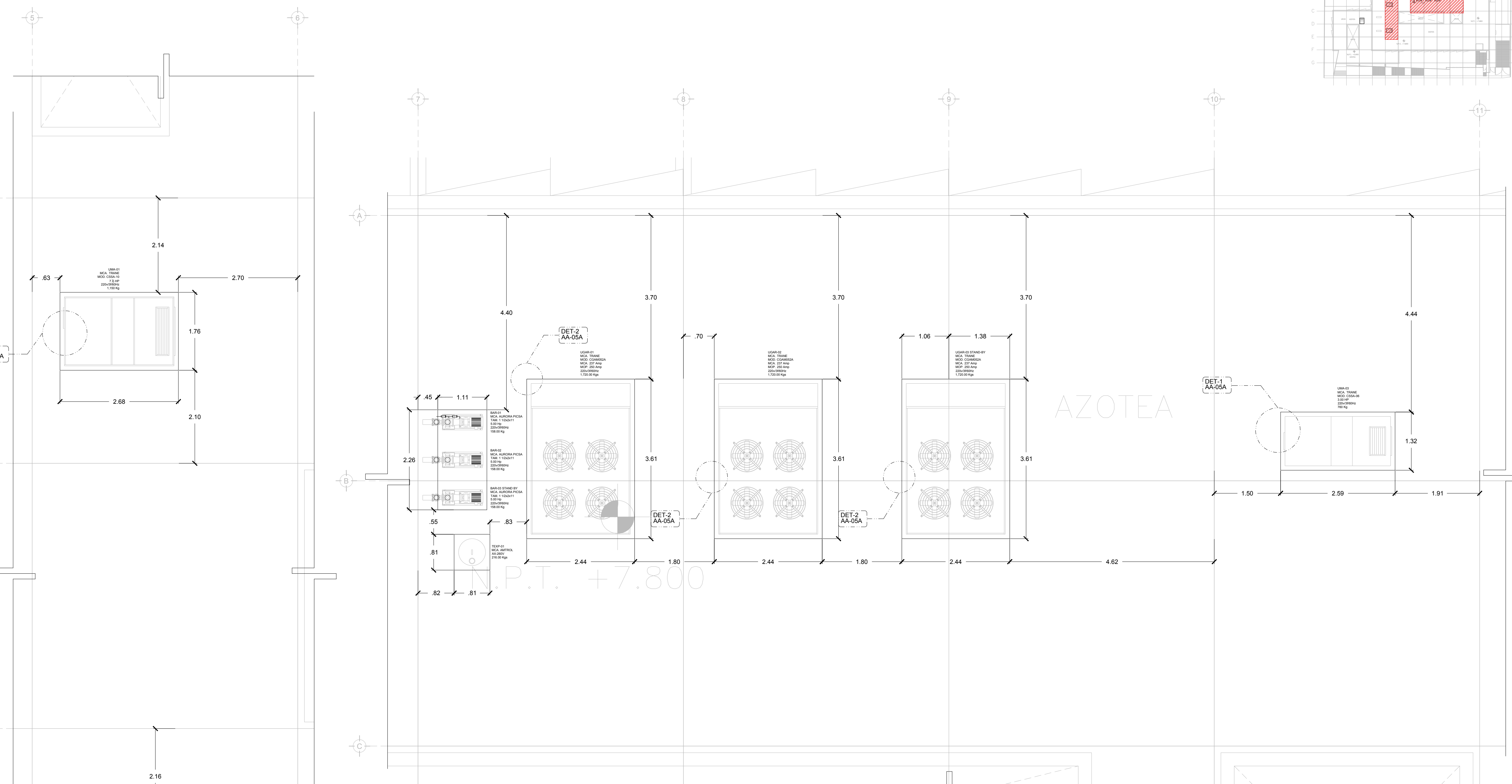
DISTRIBUCIÓN DE BASES DE EQUIPOS PLANTA AZOTEA N.L.A.L. +7.80m ESC: 1:50
