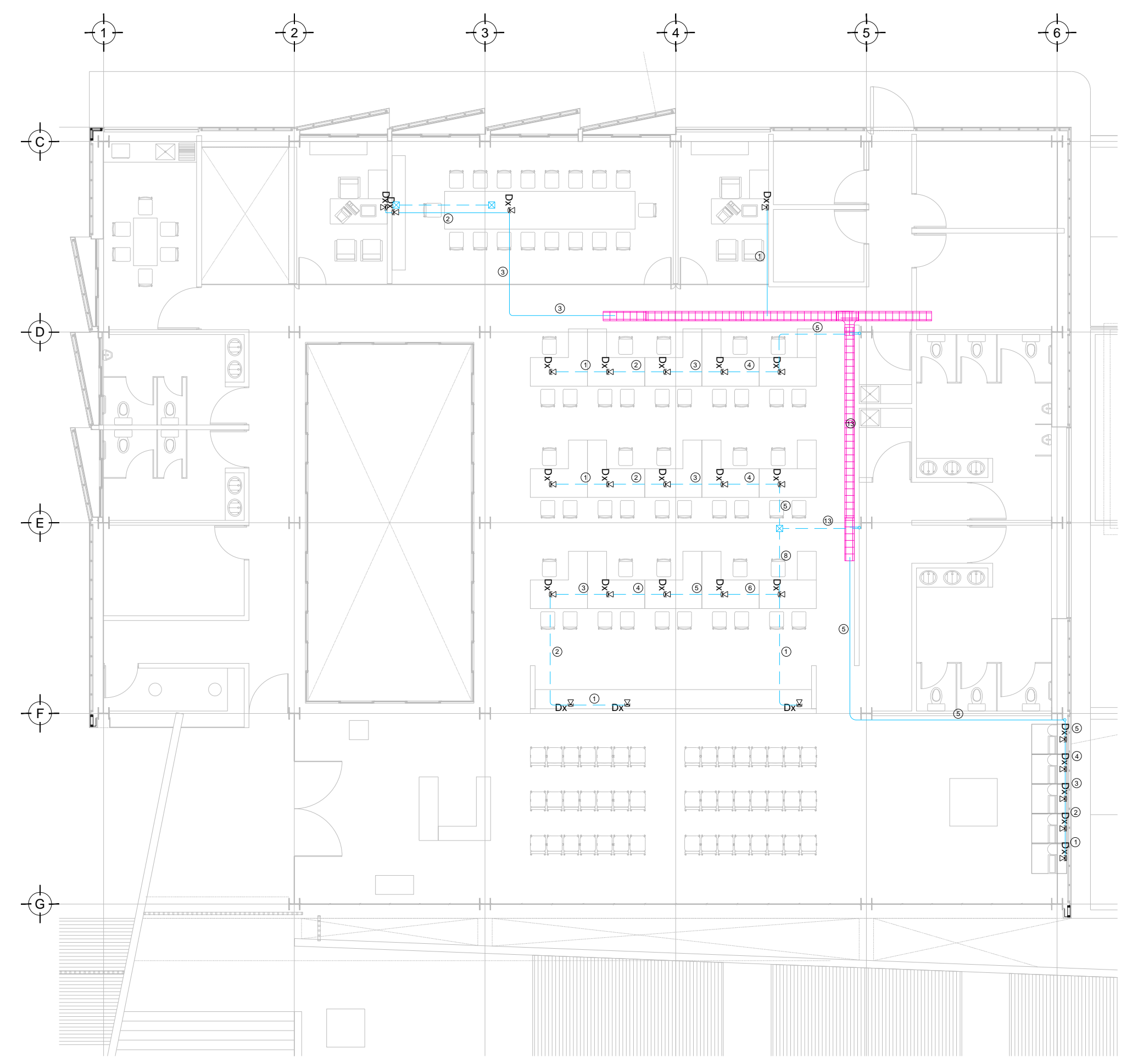
TENDIDO DE INSTALACION DE DATOS (CESI) N.P.T. ±0.00 mts. ESC: 1:125
