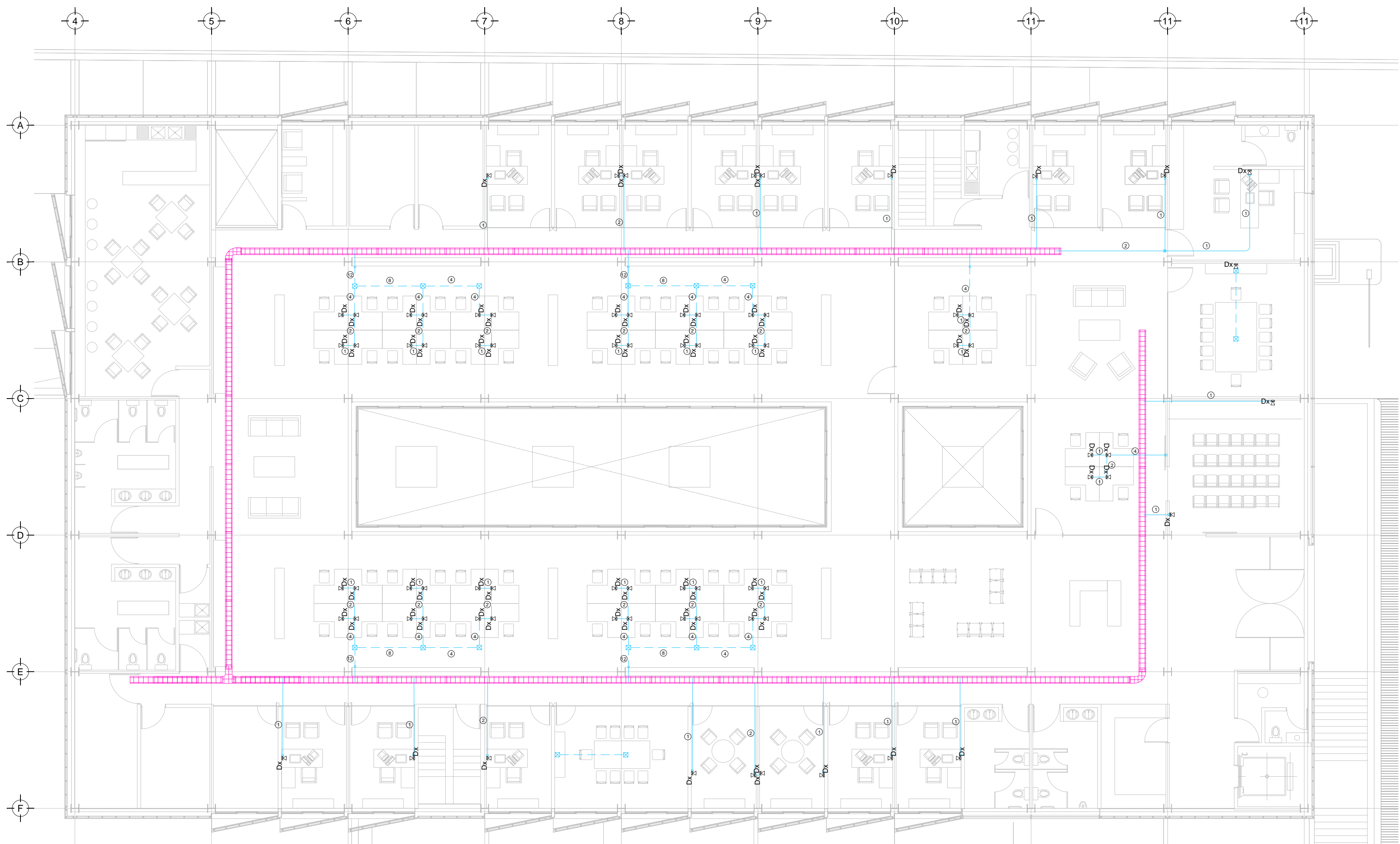
TENDIDO DE INSTALACION DE DATOS (DELEGACION) N.P.T. +3.90 ms. ESC: 1:125
