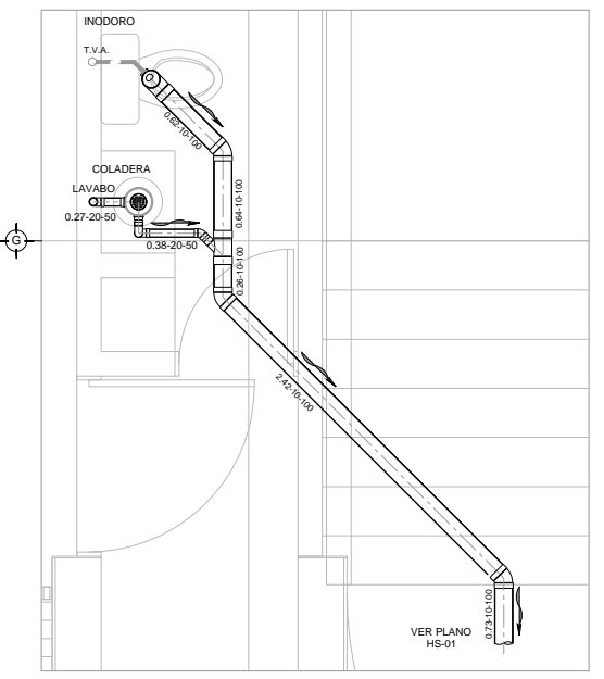
PLANTA - DISTRIBUCION - DRENAJE SANITARIO - SECCION F NIVEL ±0.00 / -1.80 ESC: 1:25
