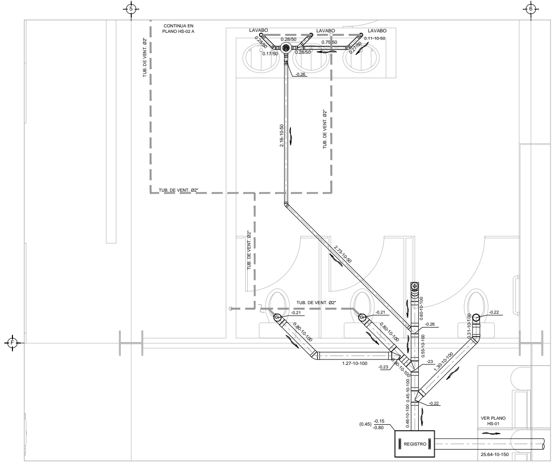
PLANTA - DISTRIBUCION - DRENAJE SANITARIO - SECCION D NIVEL ±0.00 / -1.80 ESC: 1:25
