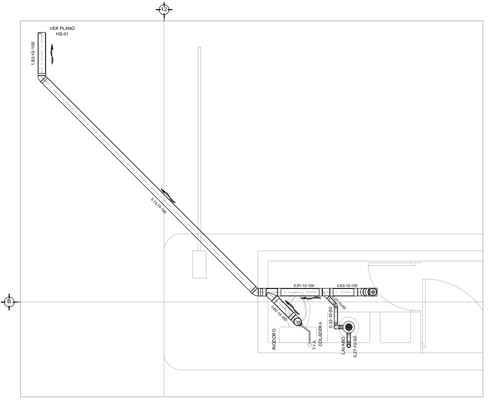
PLANTA - DISTRIBUCION - DRENAJE SANITARIO - SECCION E NIVEL ±0.00 / -1.80 ESC: 1:25
