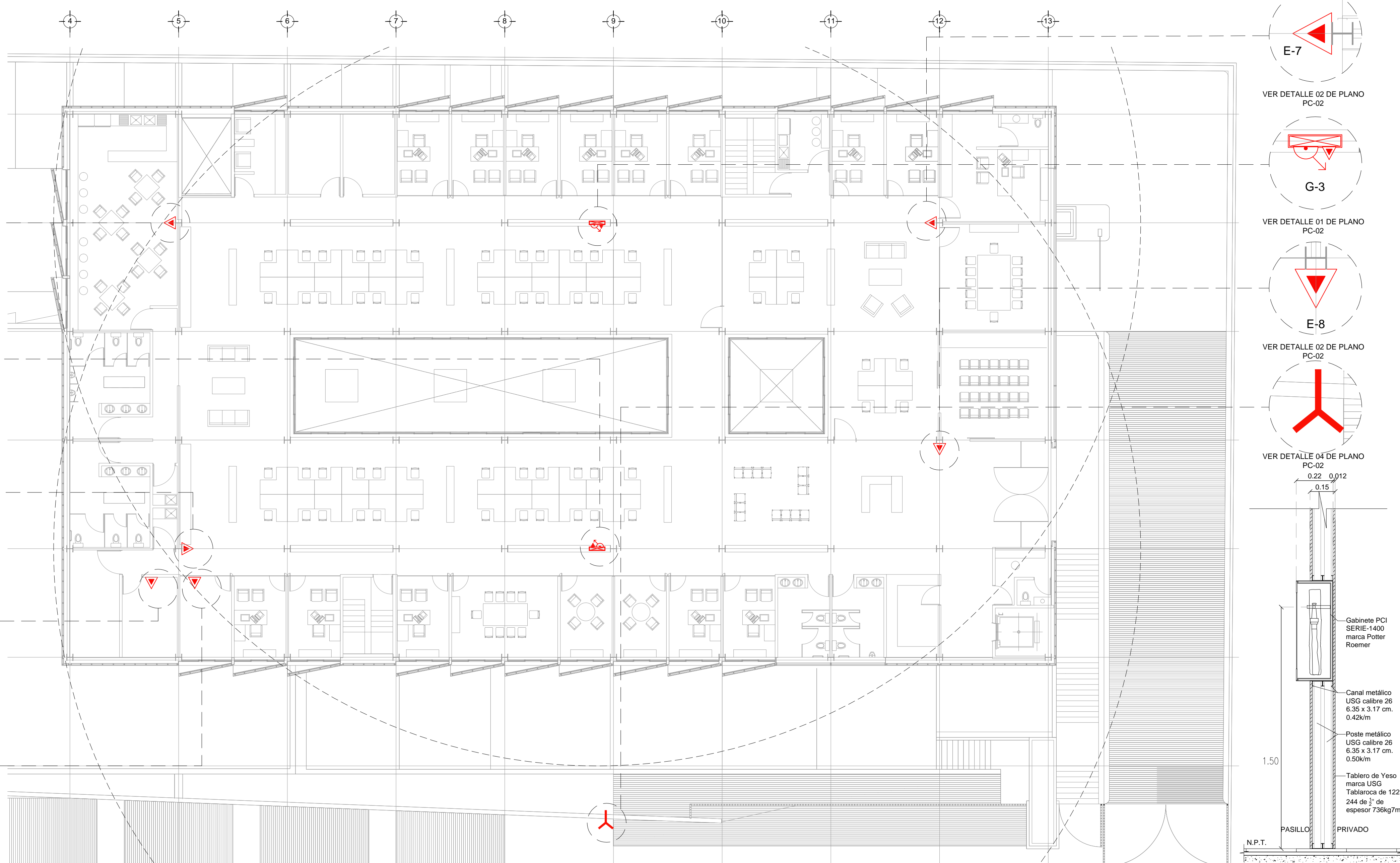
SISTEMA DE PROTECCION CONTRA INCENDIO - NIVEL +3.90 - PLANTA NIVEL 1 ESC.: 1:125
