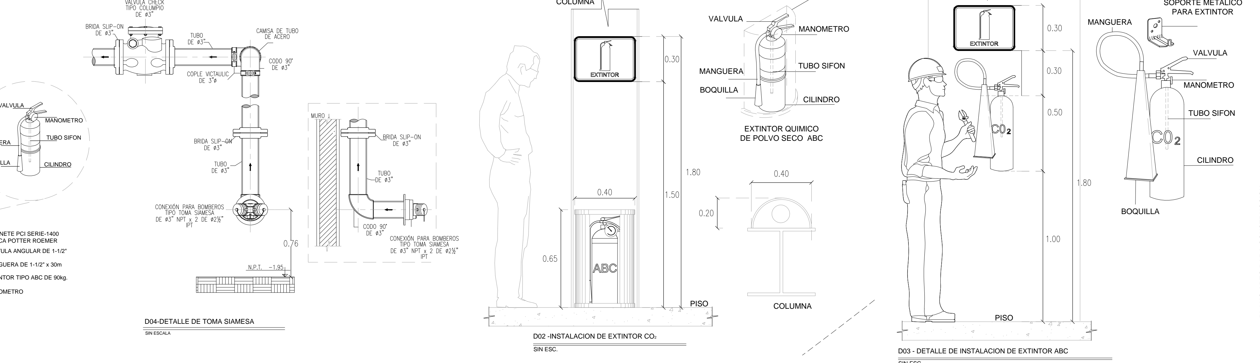
D01- DETALLE DE GABINETE SIN ESC. D02- INSTALACION DE EXTINTOR CO2 SIN ESC. D03- DETALLE DE INSTALACION DE EXTINTOR ABC SIN ESC. D04- DETALLE DE TOMA SIAMESA SIN ESC.
