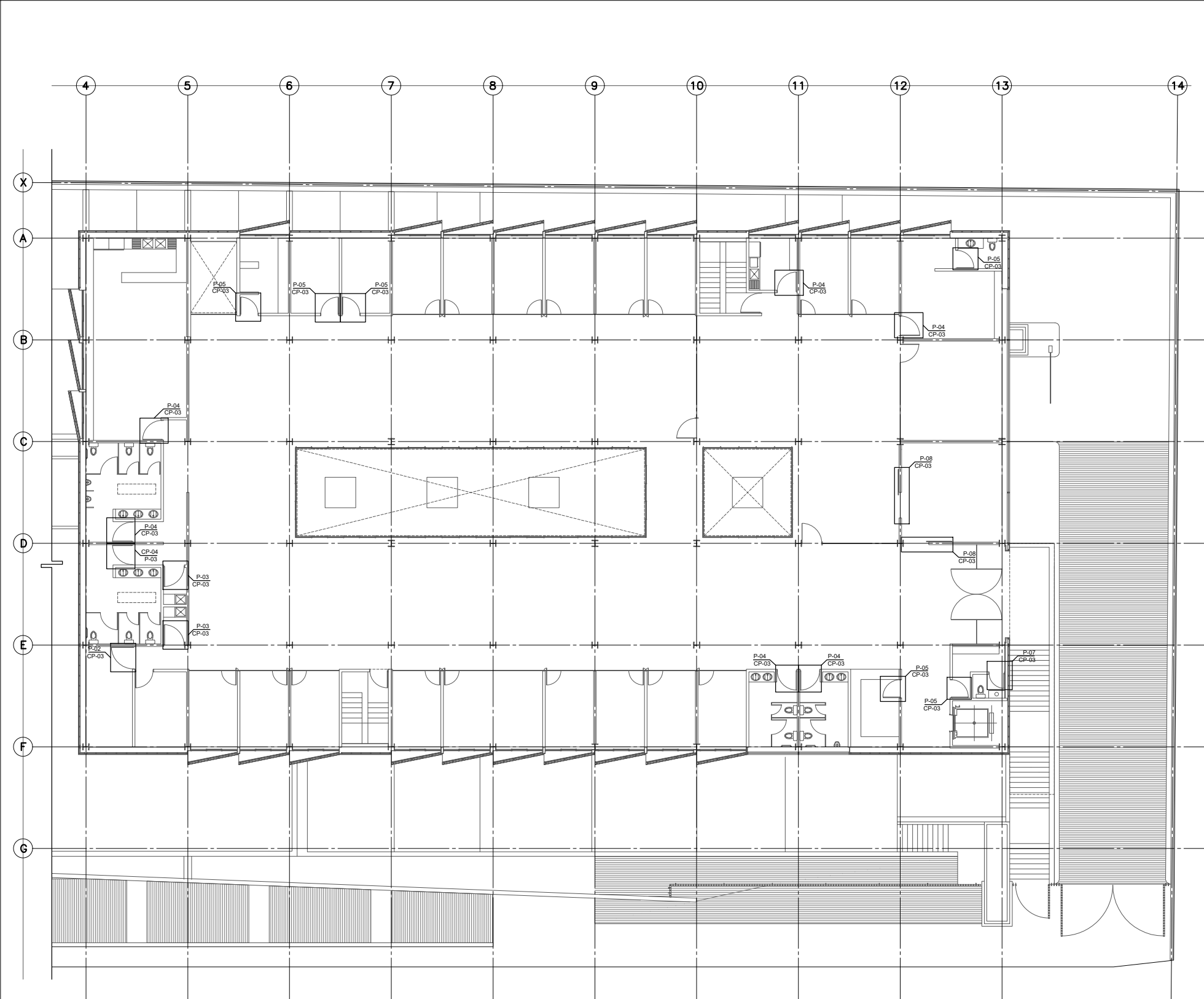
PLANTA ARQUITECTÓNICA CARPINTERÍAS N. +3.900
