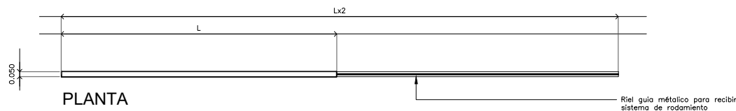
PUERTA CORREDIZA (armado tipo) ESC: 1:25
