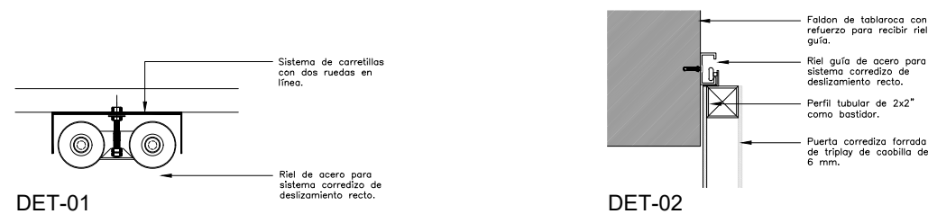
DETALLES ESC: 1:5
