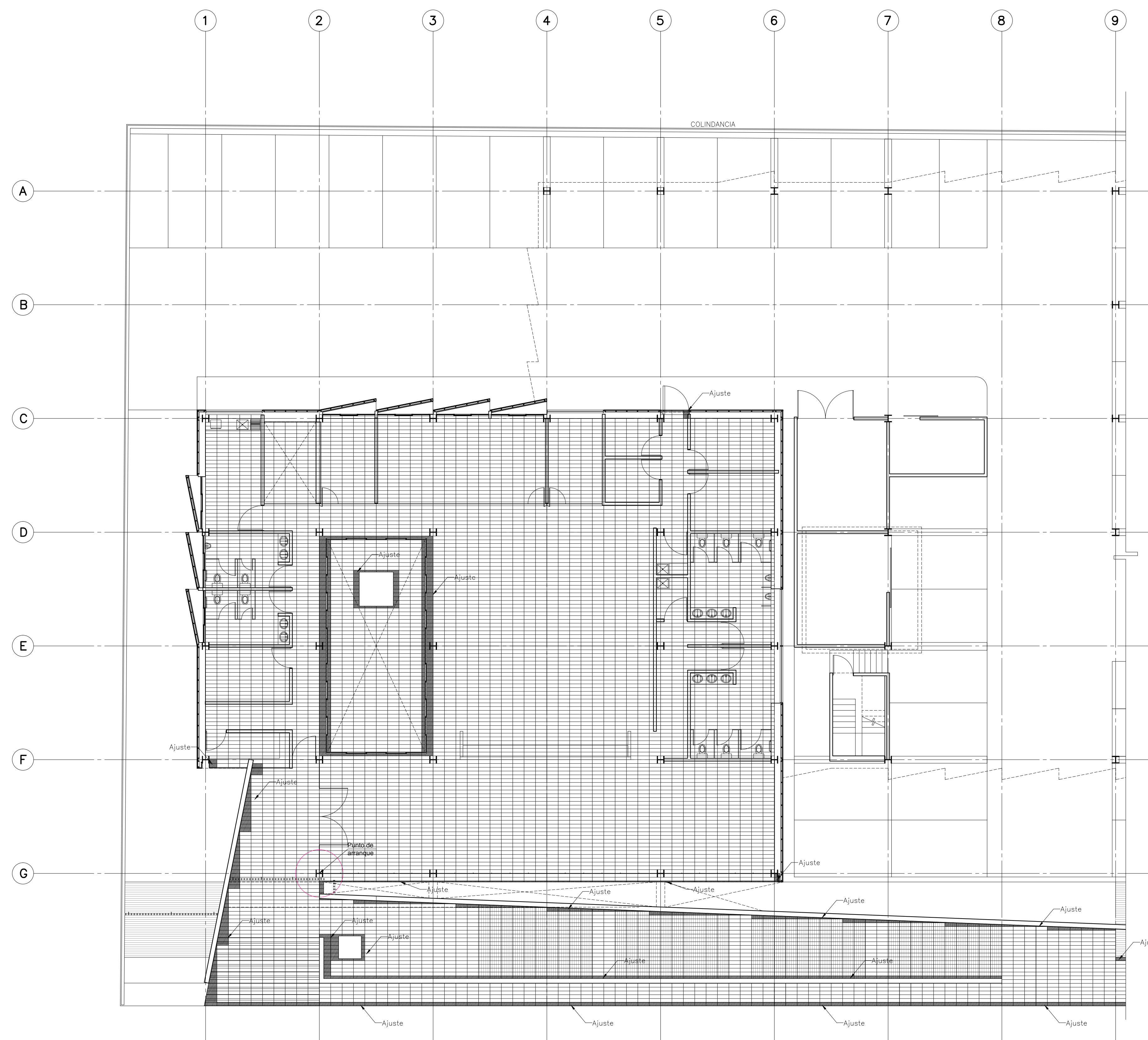
PLANTA DE DESPIECES CESI N. ±0.000
