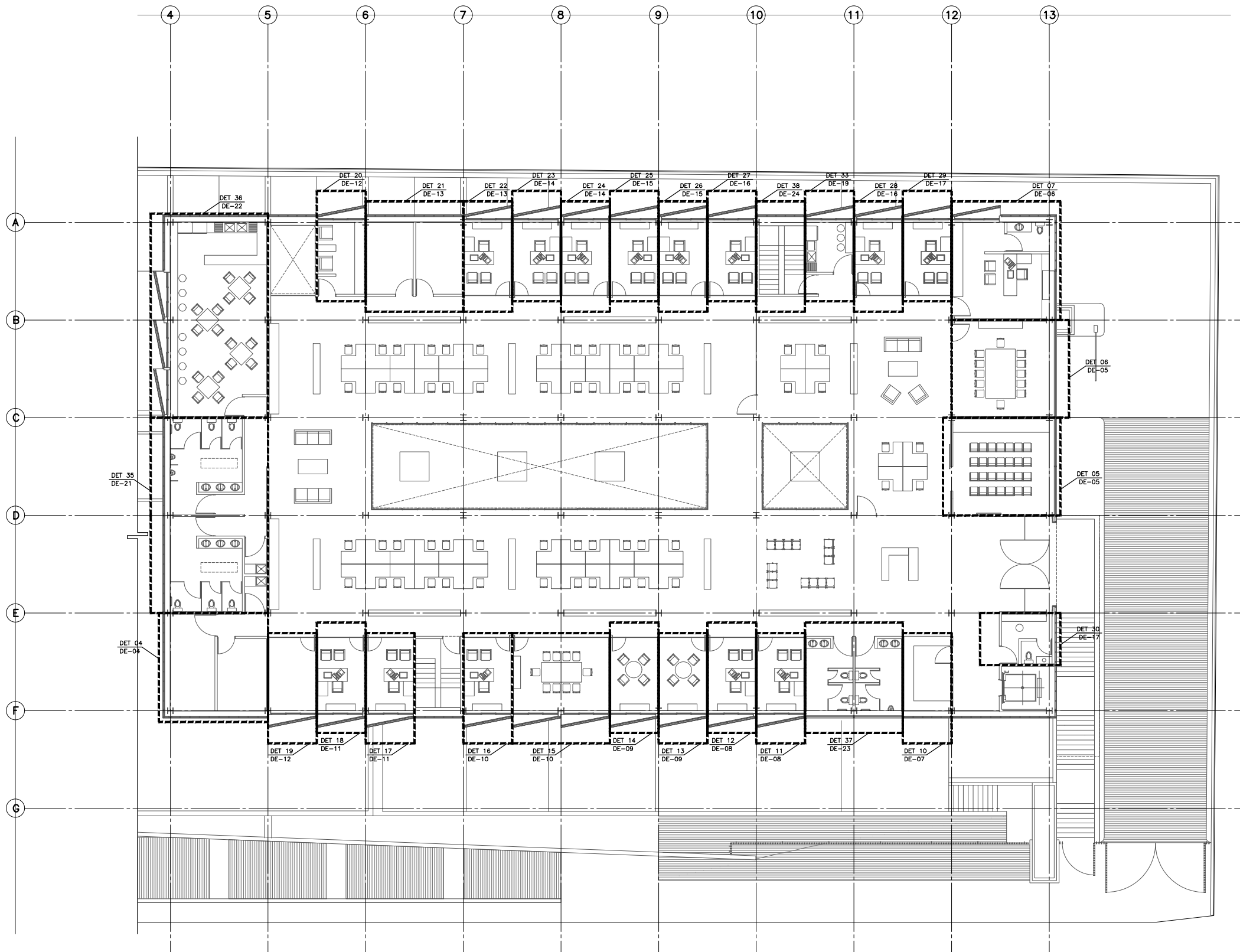
PLANTA ARQUITECTÓNICA DETALLES DELEGACIÓN N. +3.900
