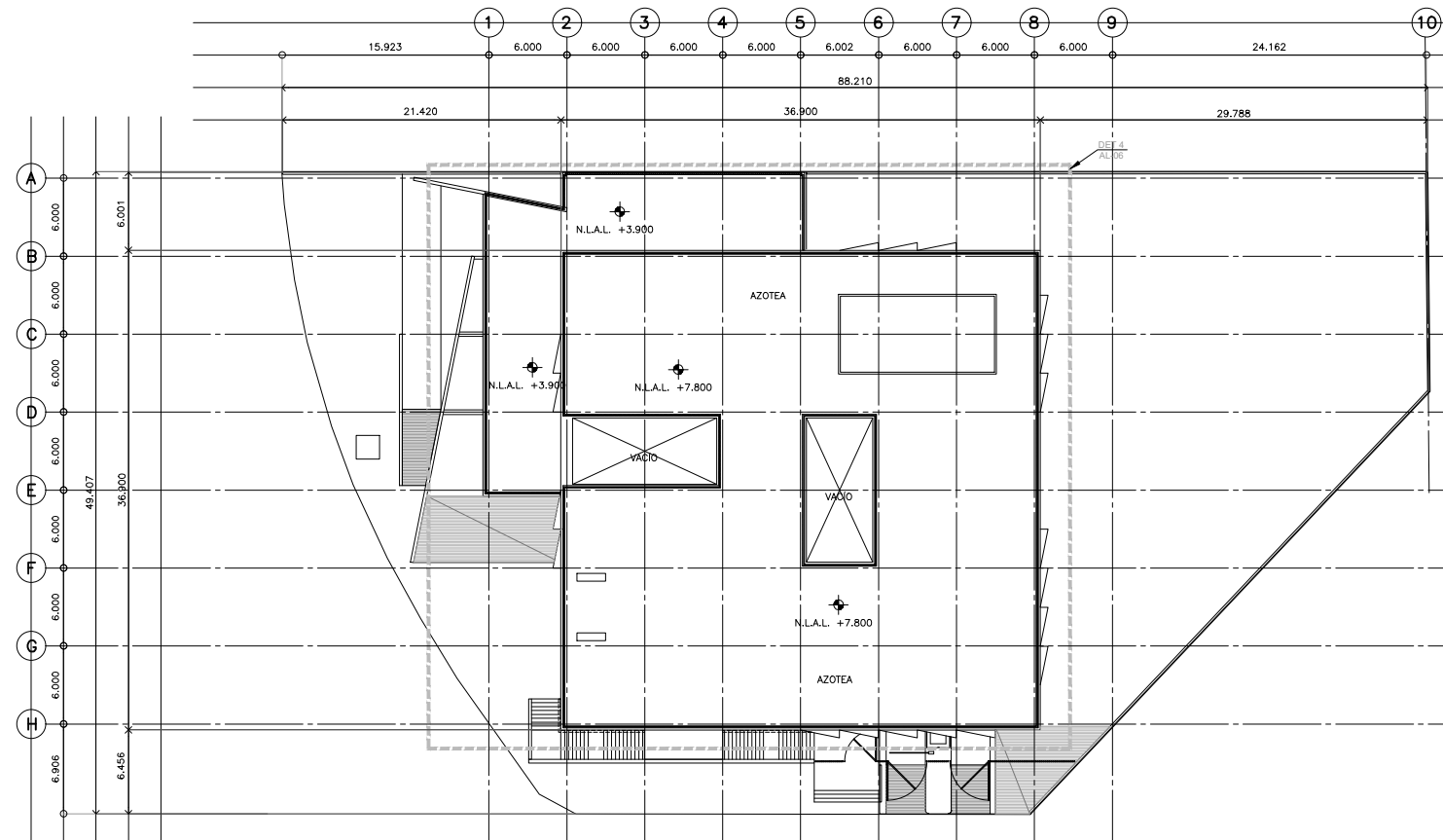
PLANTA DE AZOTEA NIVEL +7.800
