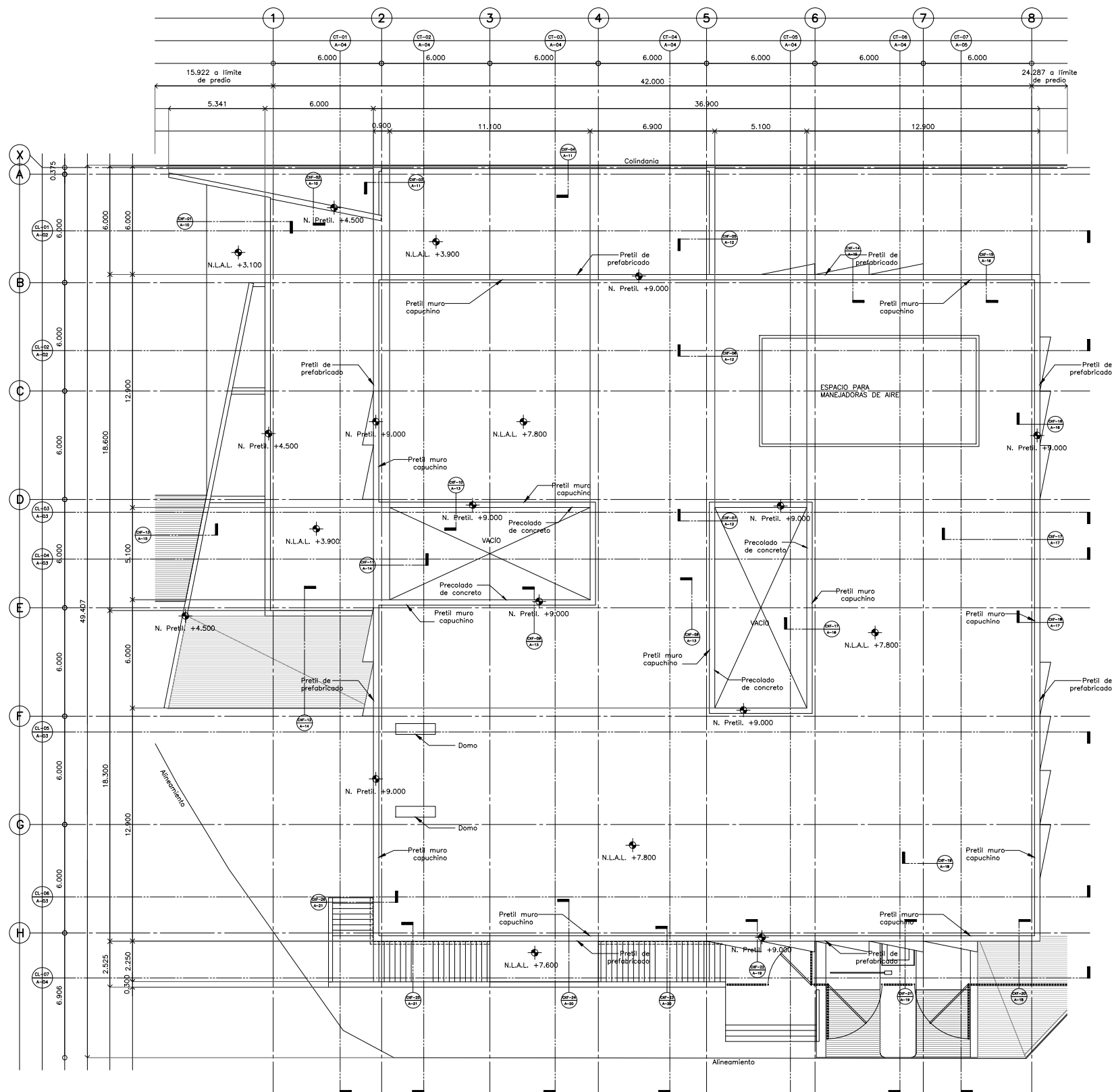
PLANTA ARQUITECTÓNICA DELEGACIÓN N. +7.800 DETALLE 4
