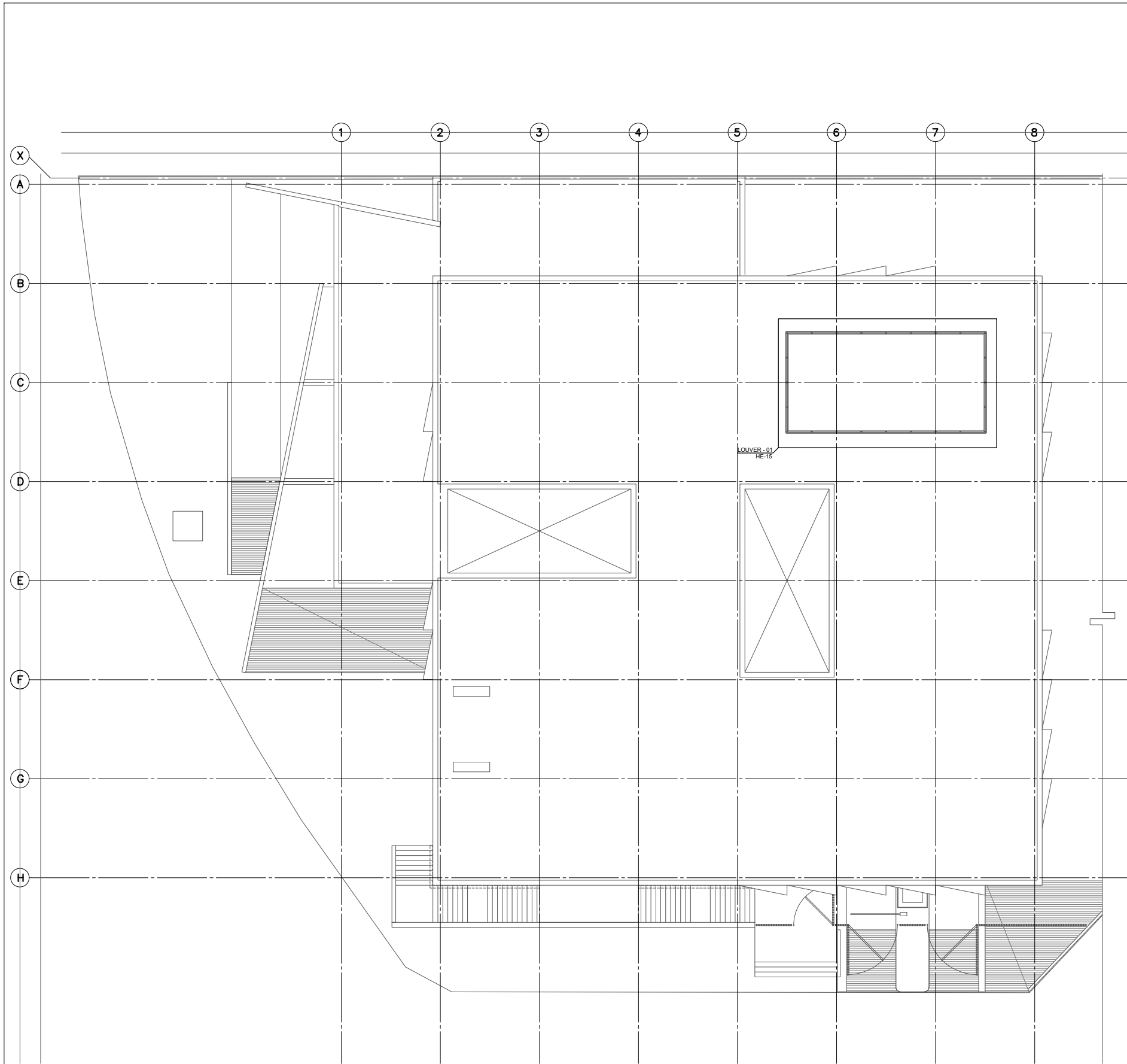
PLANTA ARQUITECTÓNICA DE HERRERÍAS NIVELES +7.800
