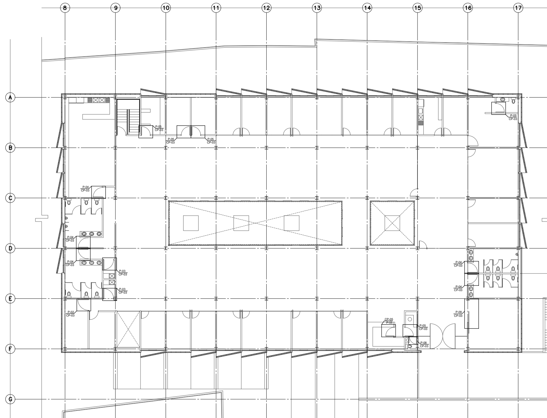
PLANTA ARQUITECTÓNICA PUERTAS LLAVE NIVEL +3.000
