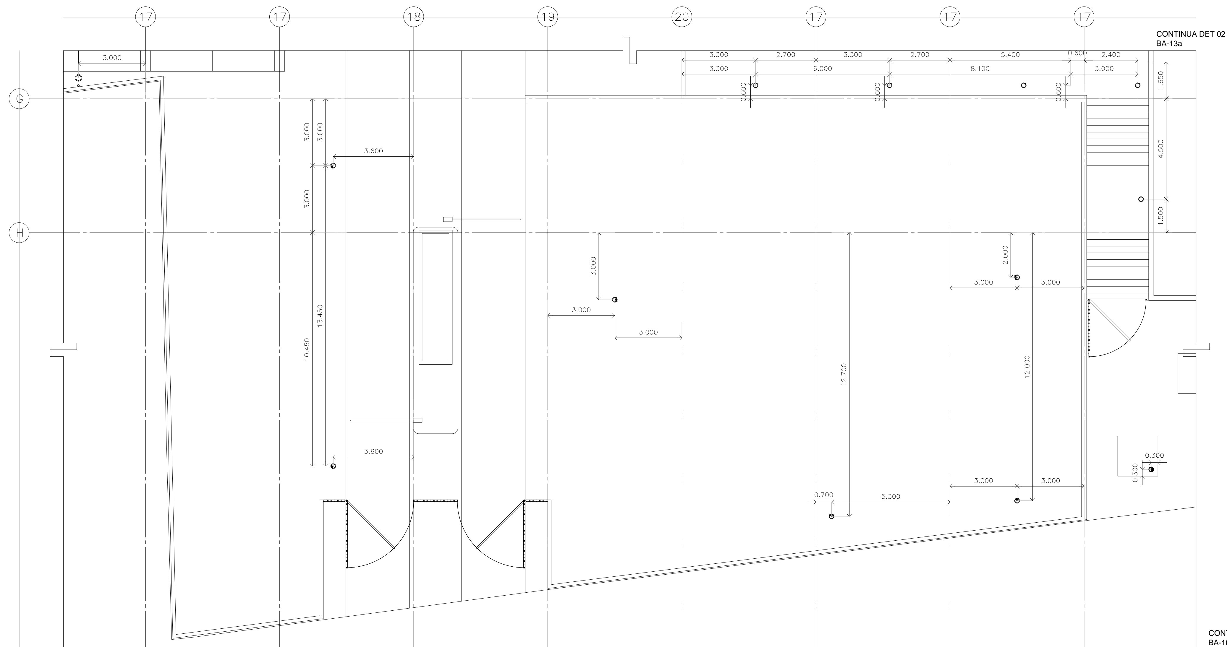
DETALLE 4 LUMINARIAS EXTERIORES CESI NIVEL ±0.000 CONTINUA DET 02 BA-13a
