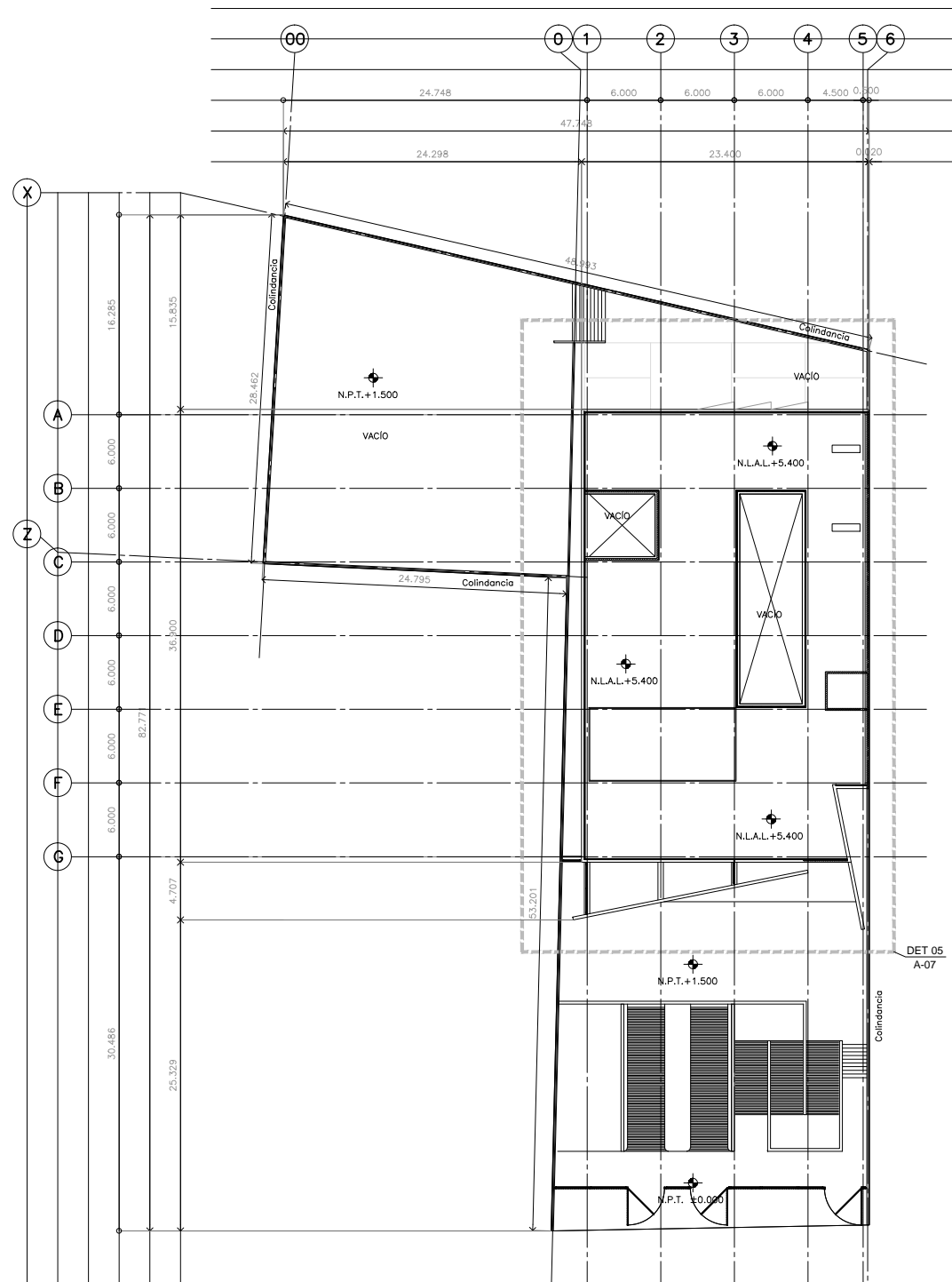
PLANTA ARQUITECTÓNICA ALBAÑILERÍAS NIVEL +5.400
