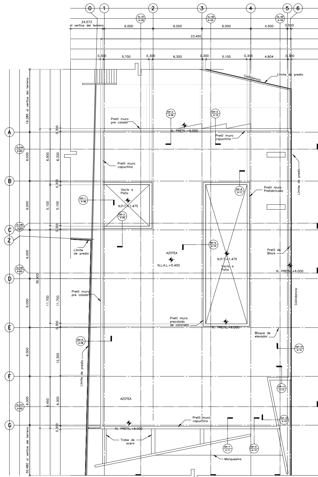
PLANTA ARQUITECTÓNICA NIVEL +5.400 DETALLE-05
