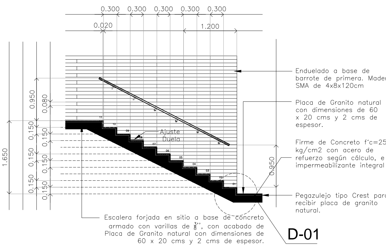
Escalera tipo 1 Sección 1
