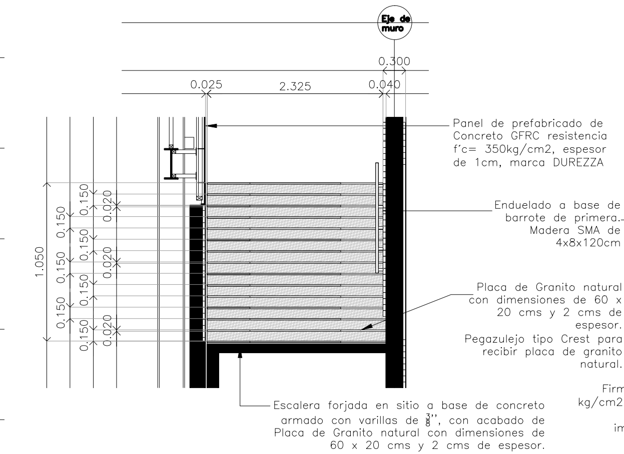
Escalera tipo 2 Alzado Escala: 1:50
