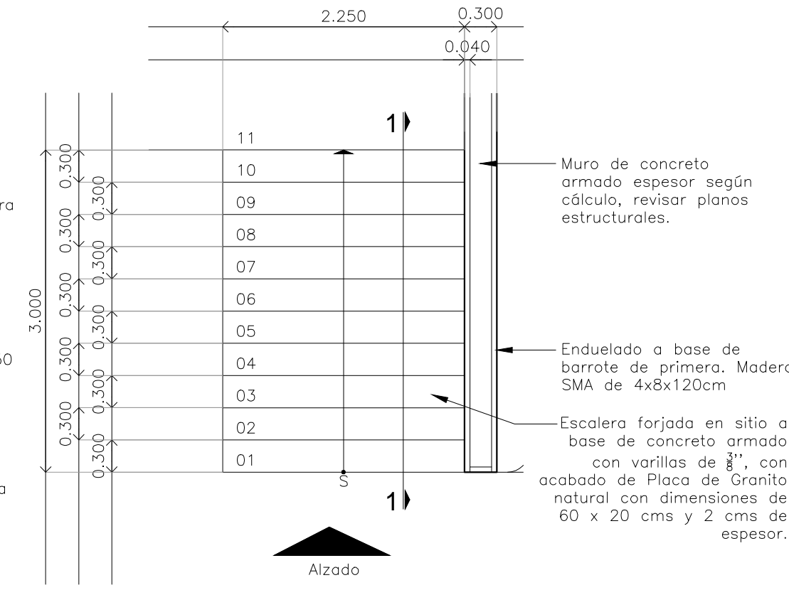
Escalera tipo 1 Planta
