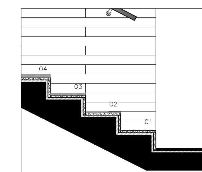
Detalle 1 Escala: 1:20
