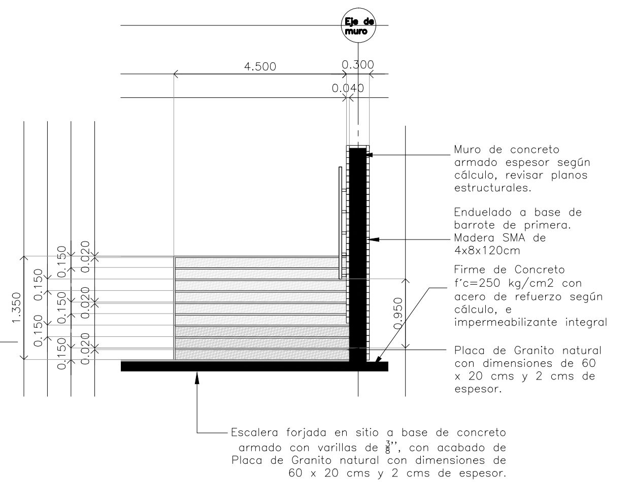
Escalera tipo 1 Alzado
