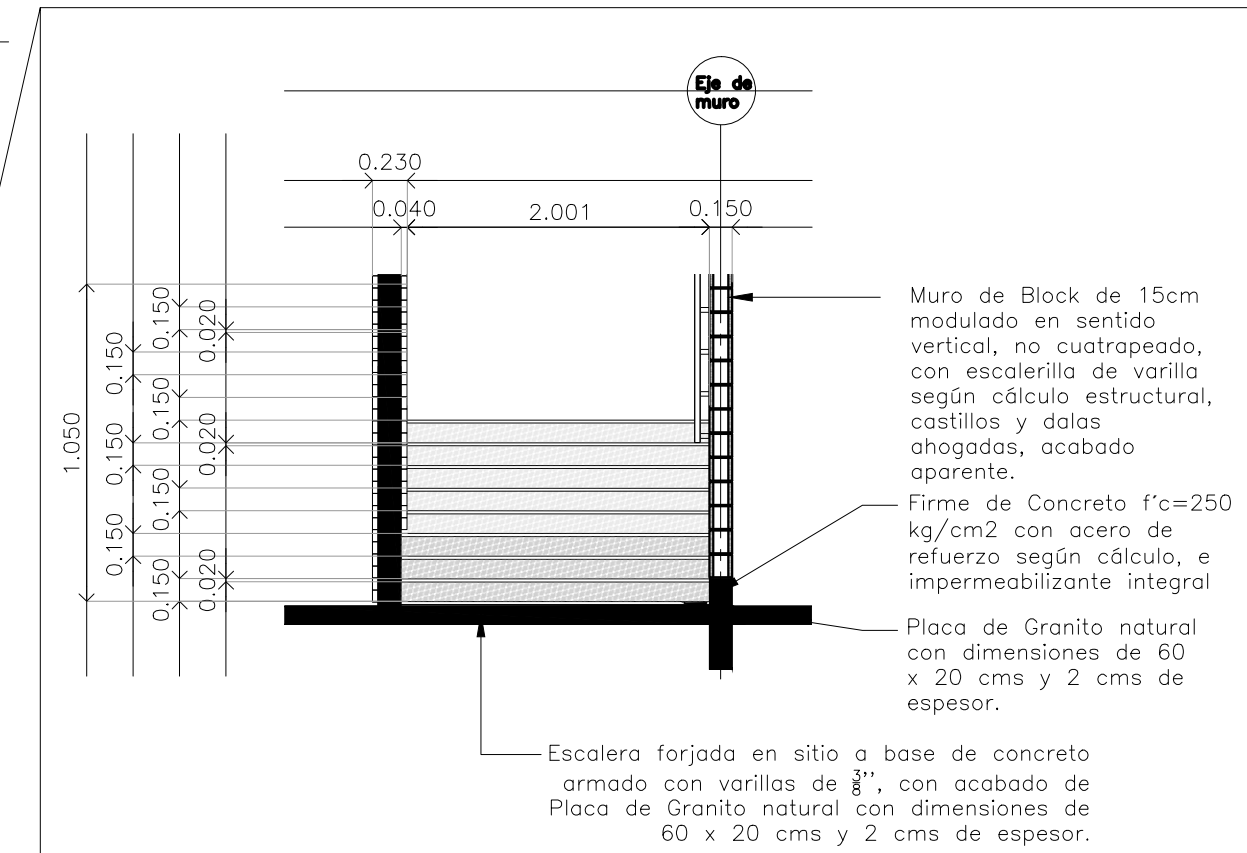
Escalera tipo 3 Alzado Escala: 1:50
