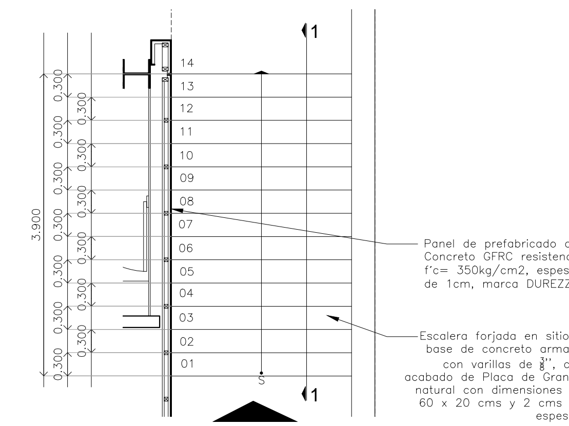
Escalera tipo 2 Planta Escala: 1:50
