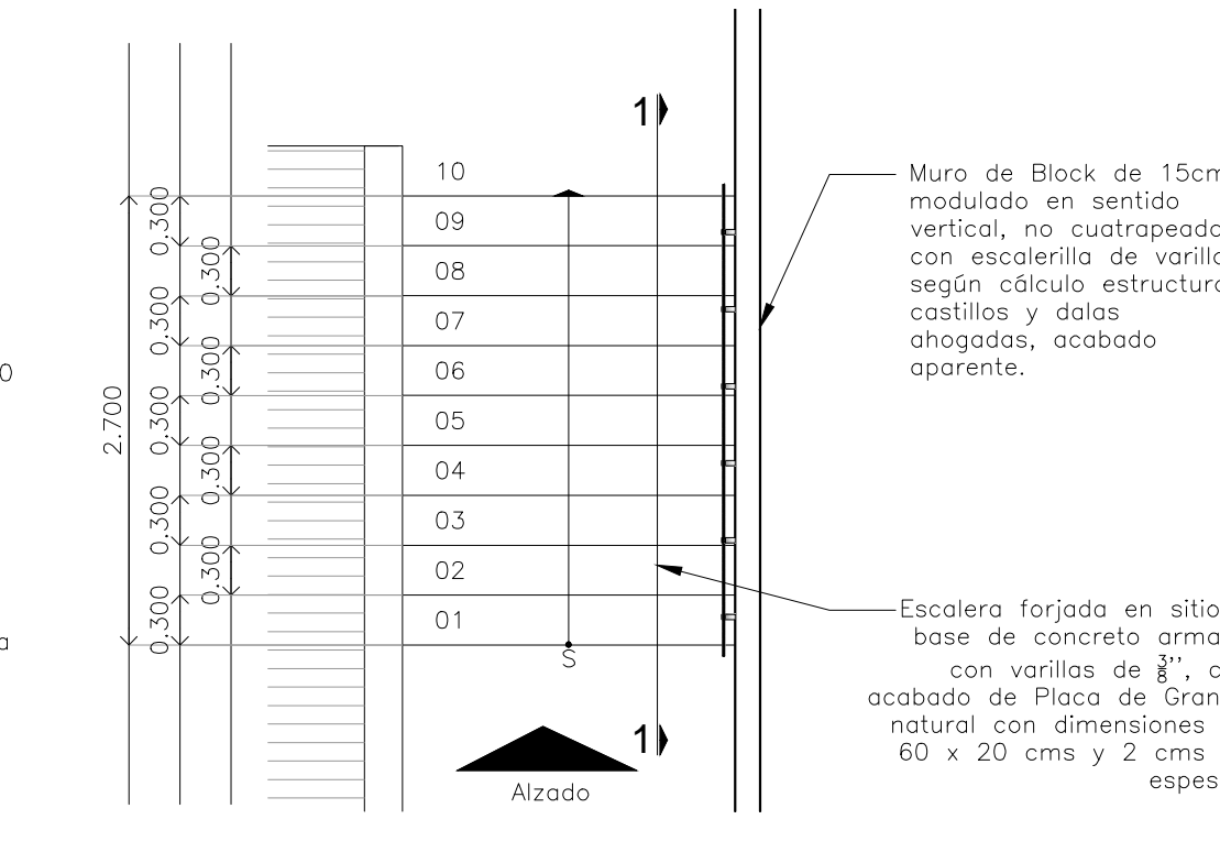
Escalera tipo 3 Planta Escala: 1:50
